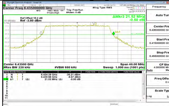
11AX20MIMO Ant2 6435
