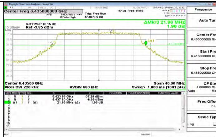
11AX20MIMO Ant1 6435
