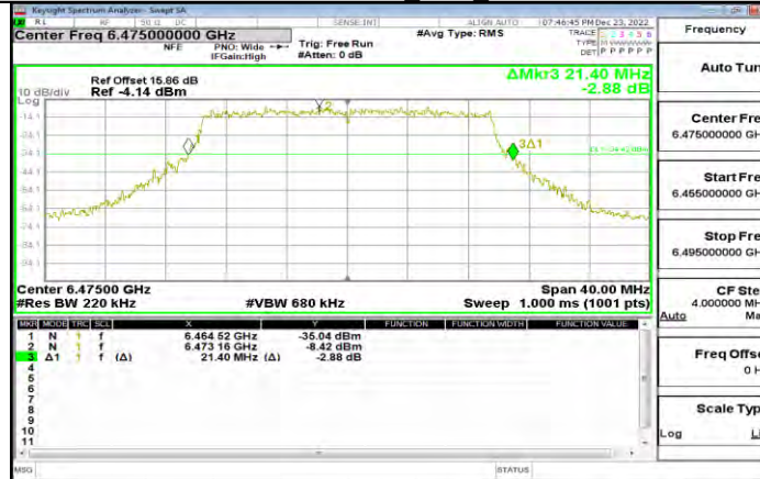
11AX20MIMO Ant1 6475
