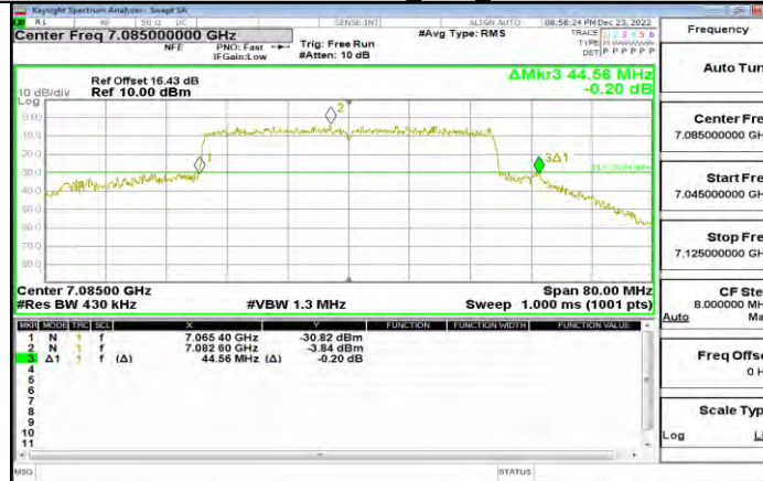
11AX40MIMO_Ant1_7085
