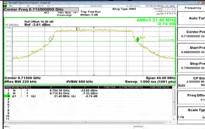
11AX20MIMO Ant1 6715
