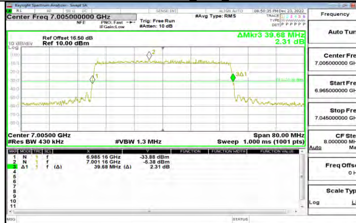
11AX40MIMO_Ant2_7005
