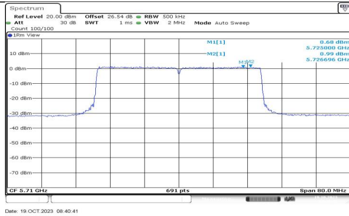
11AX40MIMO_Ant4_5710_UNII-3
