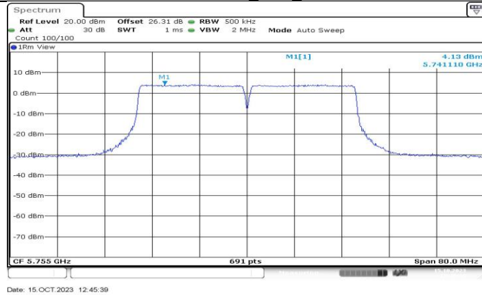
11N40MIMO Ant4 5755
