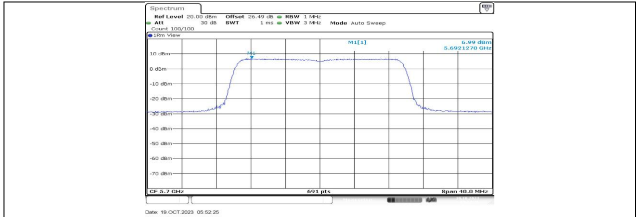
11AX20MIMO_Ant4_5700
