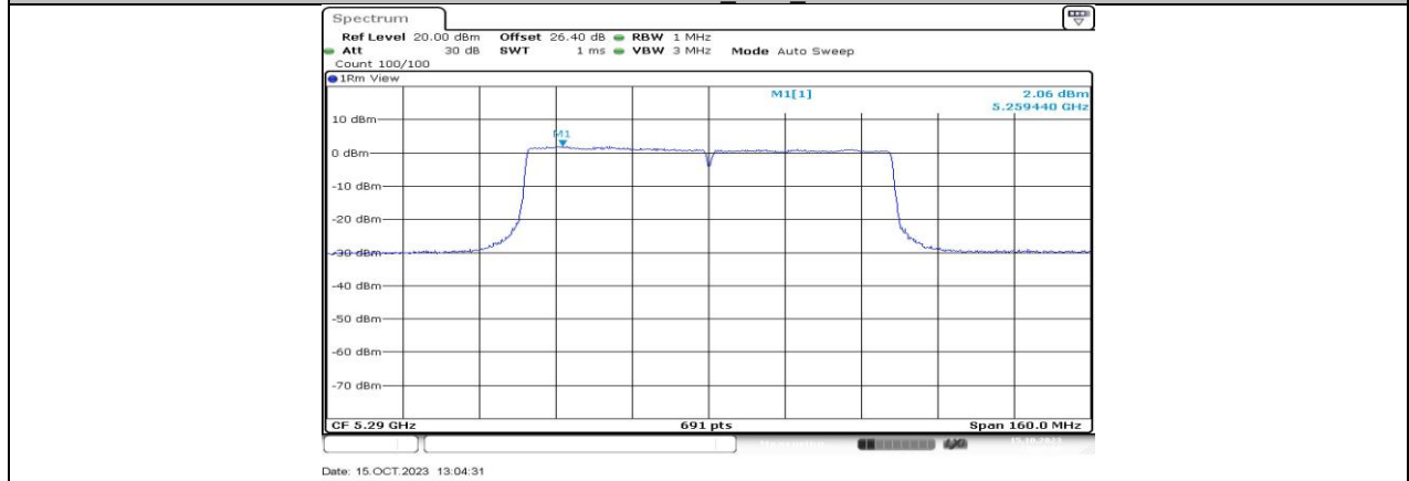
11AC80MIMO_Ant4_5290
