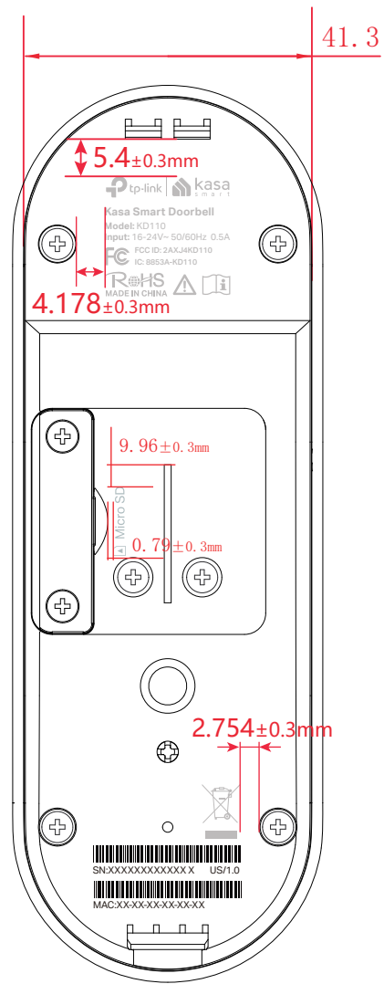
尺寸图
