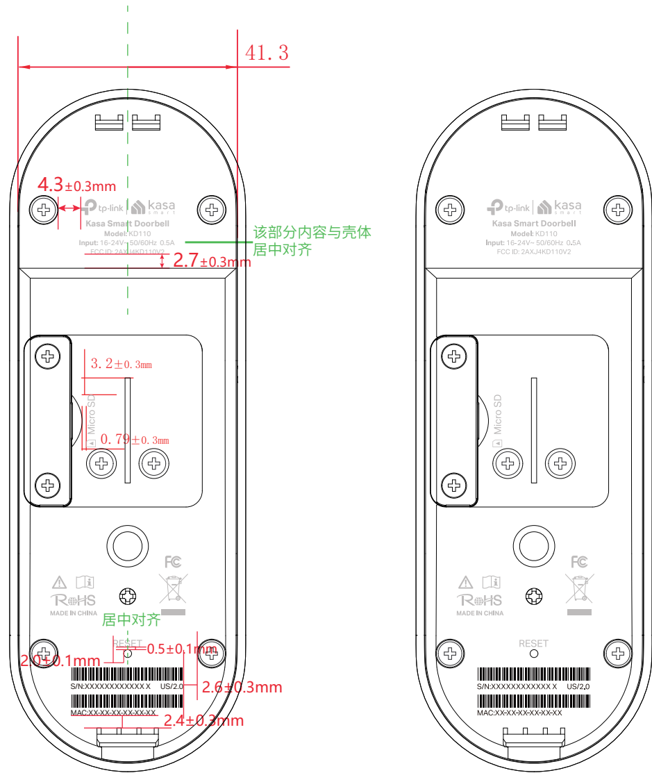
尺寸图
