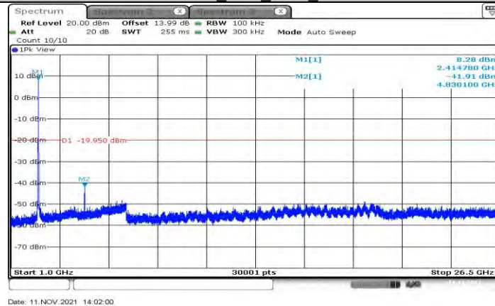
11N20SISO Ant1 2417 1000~26500
