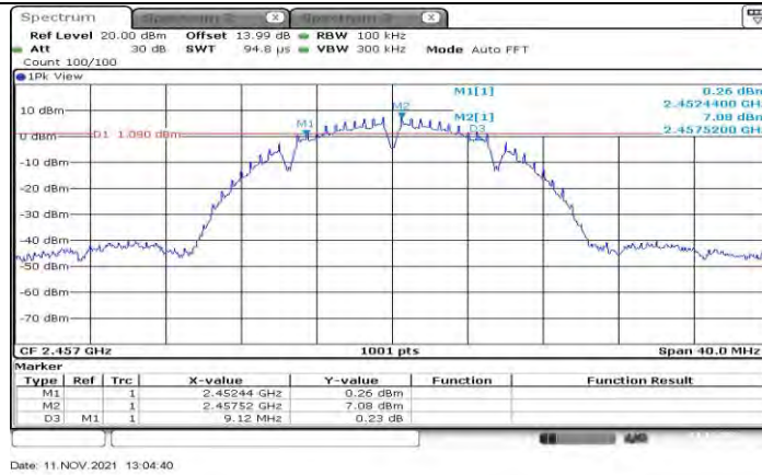
11B Ant1 2457
