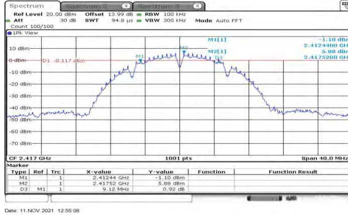
11B Ant1 2417
