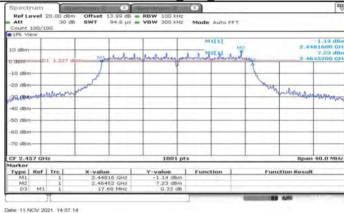
11N20SISO Ant1 2457
