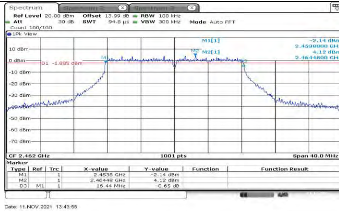
11G Ant1 2462
