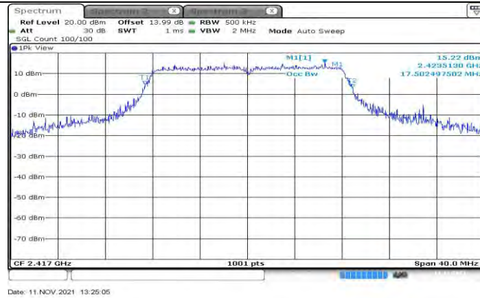
11G Ant1 2417
