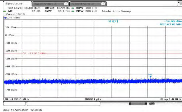
11B_Ant1_2417_30~1000
