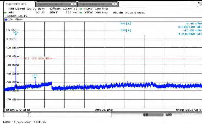
11G_Ant1_2457_1000~26500
