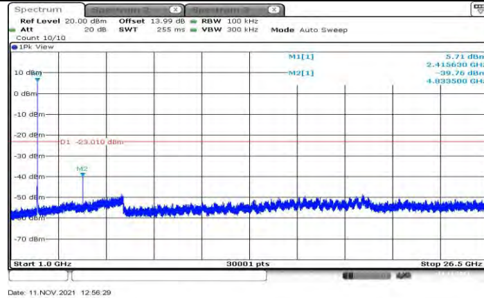
11B_Ant1_2417_1000~26500
