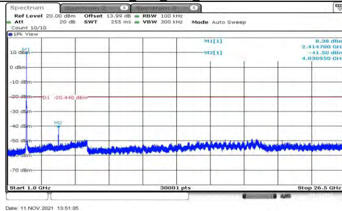
11G_Ant1_2417_1000~26500
