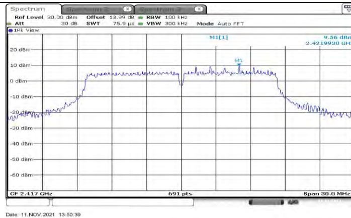
11G_Ant1_2417_0~Reference
