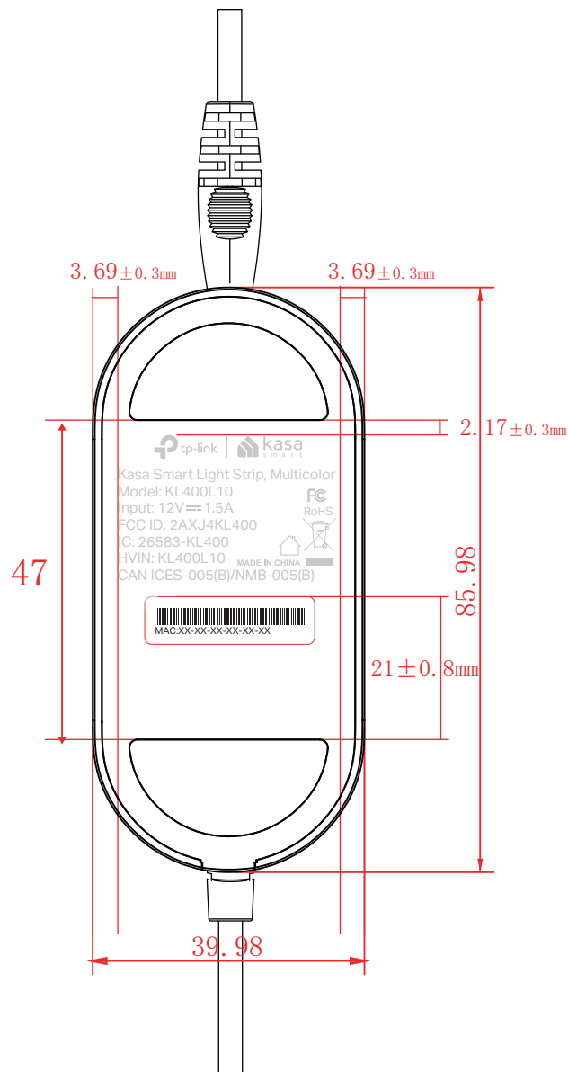
尺寸图
