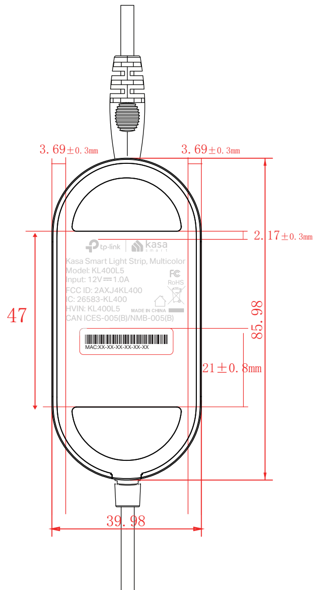
尺寸图
