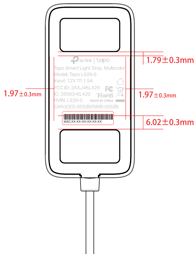
尺寸图
