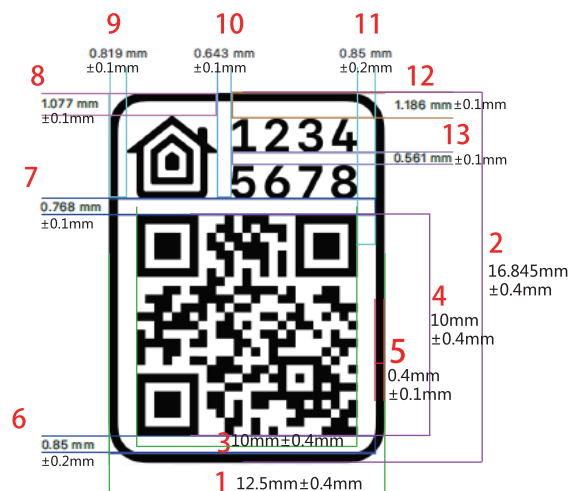
尺寸图
