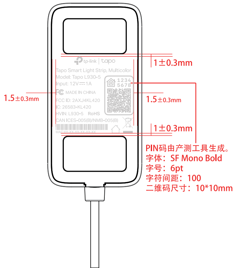
尺寸图
