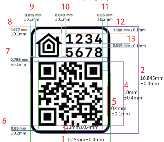
尺寸图
