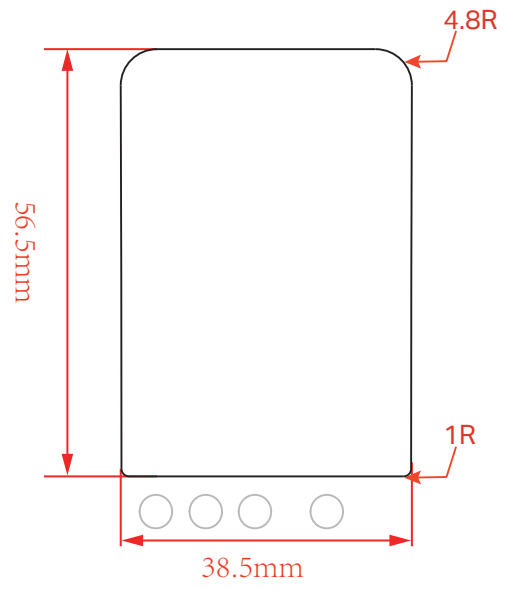
尺寸图
