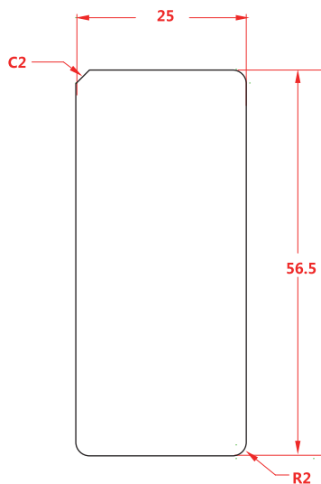
尺寸图
