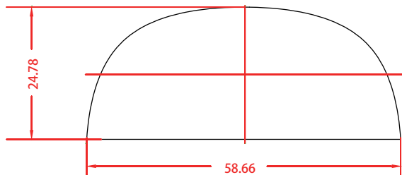
结构尺寸图
