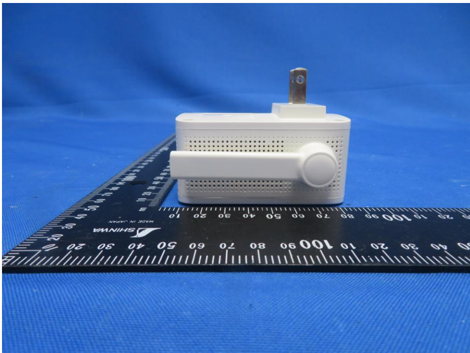
(4) EUT Photo
