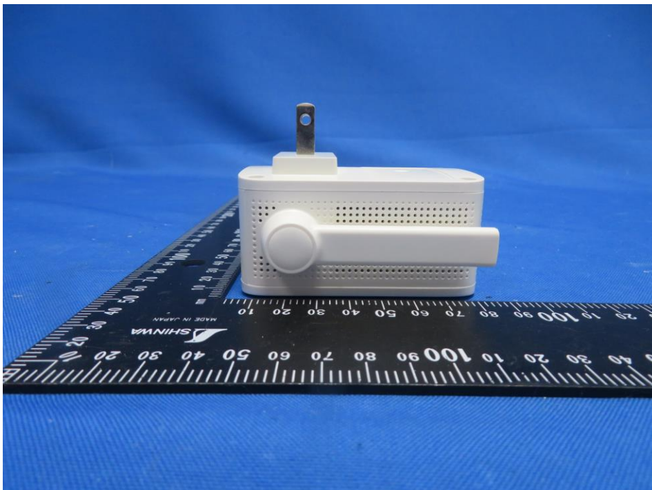
(6) EUT Photo
