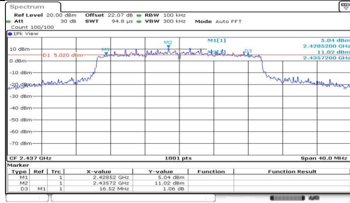
11AX20MIMO_Ant2_2437
