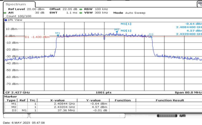
11AX40MIMO_Ant2_2427
