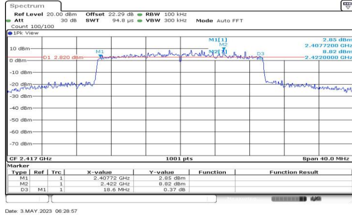
11AX20MIMO_Ant4_2417
