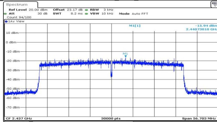
11AX40MIMO_Ant2_2437
