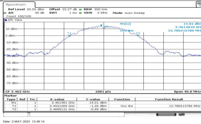
11B-CDD_Ant4_2462
