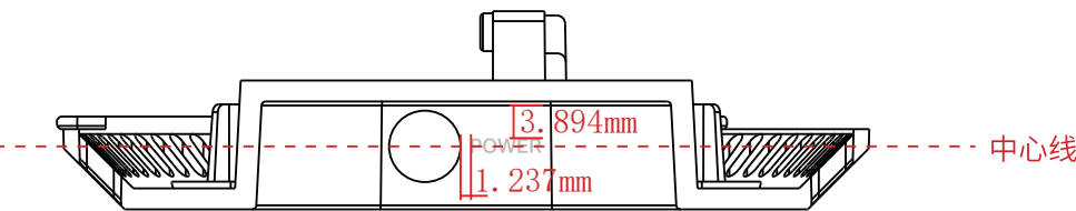
Power接口icon尺寸图
