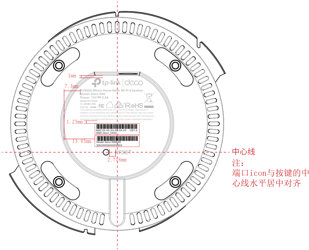
底壳镭雕尺寸图
