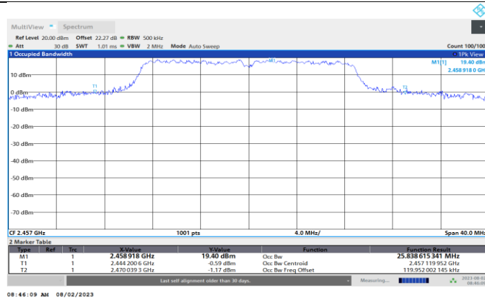
11N20MIMO_Ant4_2457
