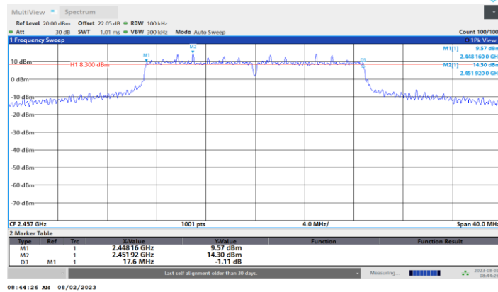
11N20MIMO_Ant2_2457
