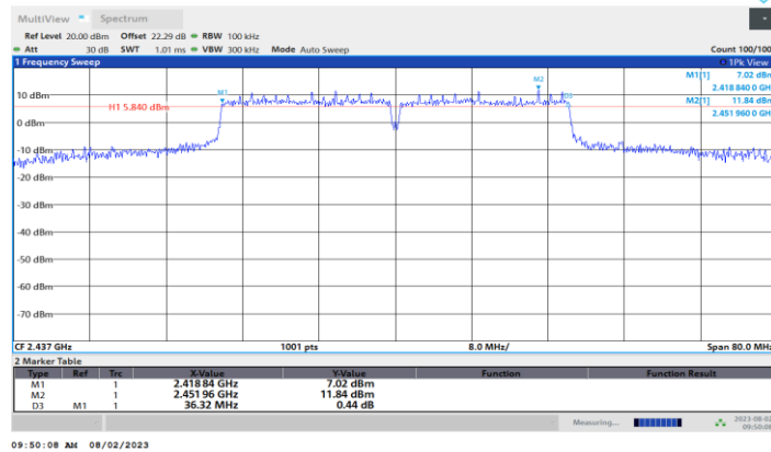
11N40MIMO_Ant4_2437
