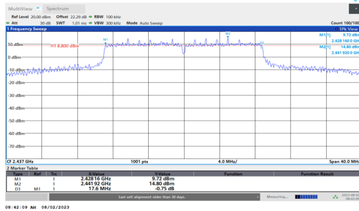
11N20MIMO_Ant4_2437
