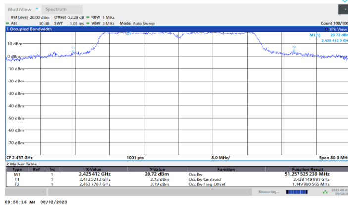
11N40MIMO_Ant4_2437
