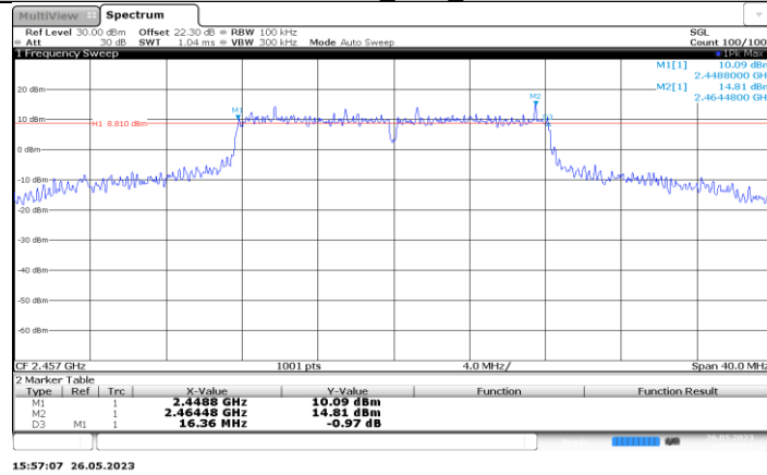
11G-CDD_Ant4_2457
