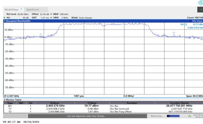
11N20MIMO_Ant4_2437
