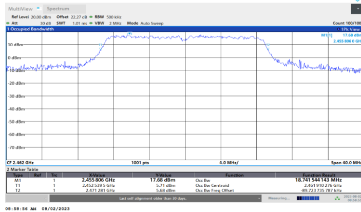
11N20MIMO_Ant4_2462
