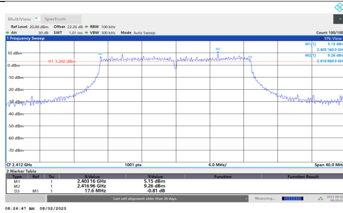
11N20MIMO_Ant4_2412
