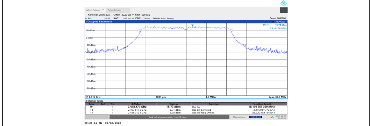
11N20MIMO_Ant4_2417
