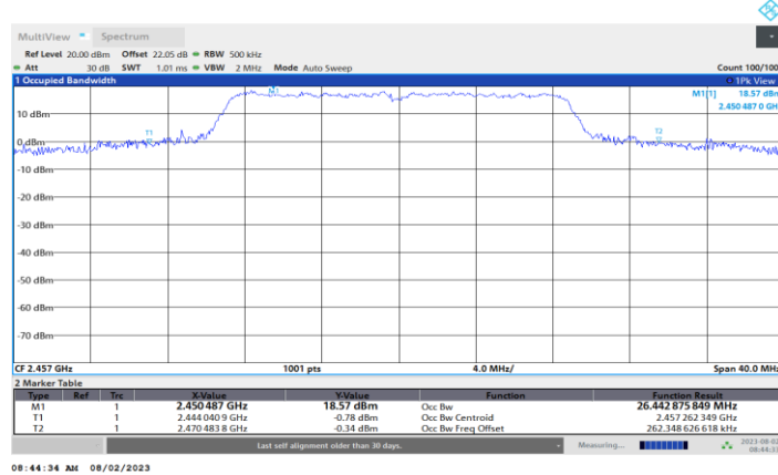
11N20MIMO_Ant2_2457
