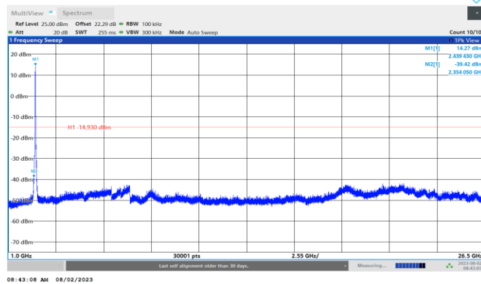
11N20MIMO_Ant4_2437_1000~26500
