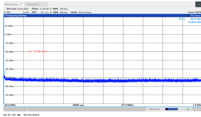
11N40MIMO_Ant4_2447_30~1000
