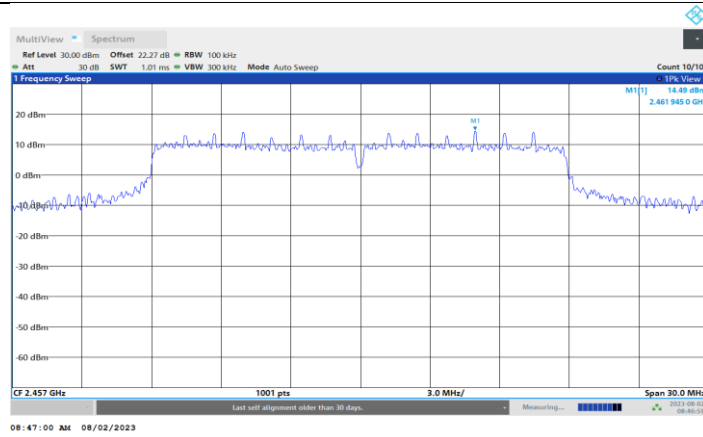
11N20MIMO_Ant4_2457_0~Reference
