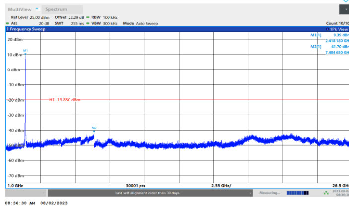
11N20MIMO_Ant4_2417_1000~26500
