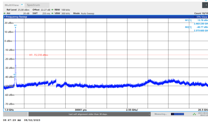
11N20MIMO_Ant4_2457_1000~26500
