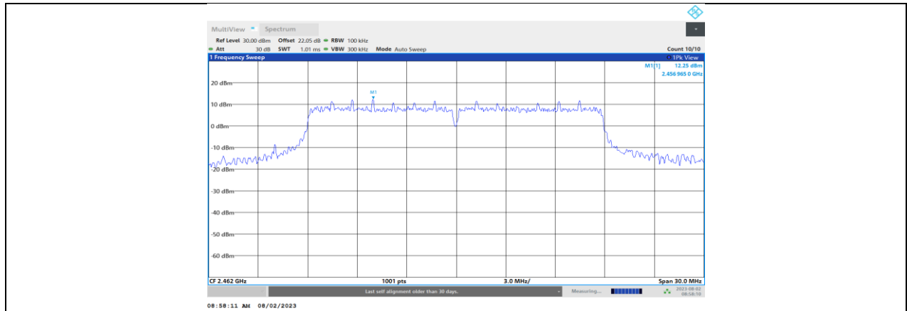
11N20MIMO_Ant2_2462_0~Reference
