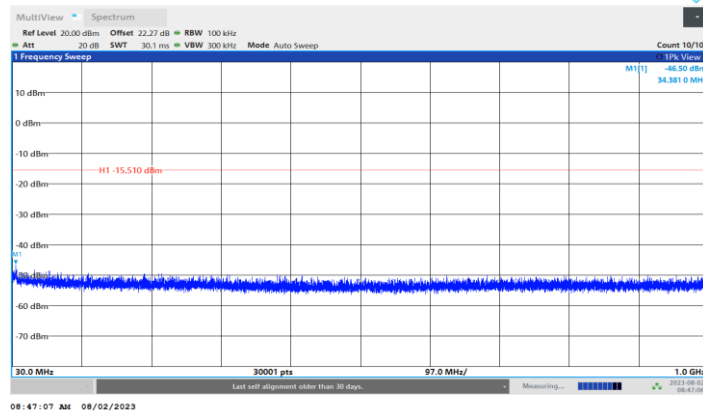
11N20MIMO_Ant4_2457_30~1000
