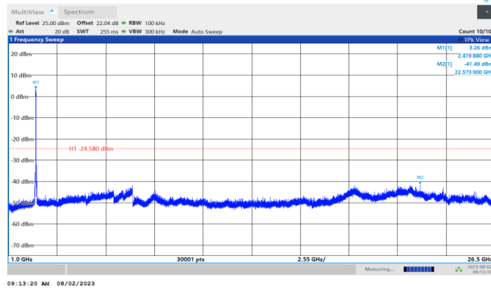
11N40MIMO_Ant2_2422_1000~26500
