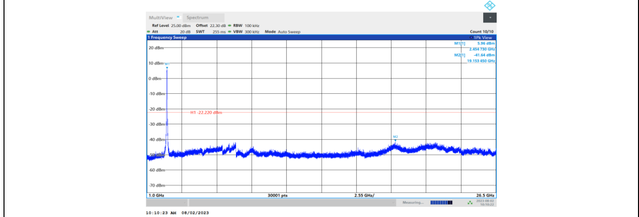
11N40MIMO_Ant4_2452_1000~26500
