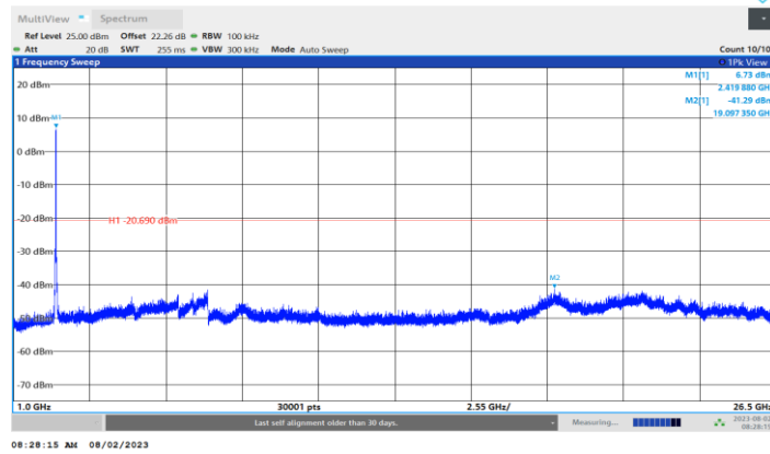
11N20MIMO_Ant4_2412_1000~26500
