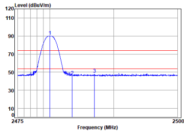
Left BT_DH5_TX_CH_78_Horizontal
