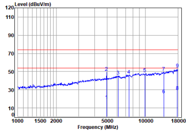
Left BT_DH5_TX_CH_78_Horizontal
