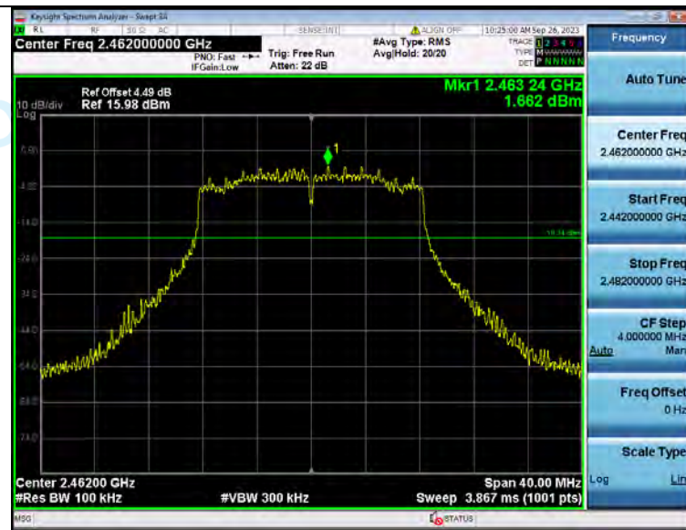
2 Bandedge NVNT ANT1 802 11g 2462
