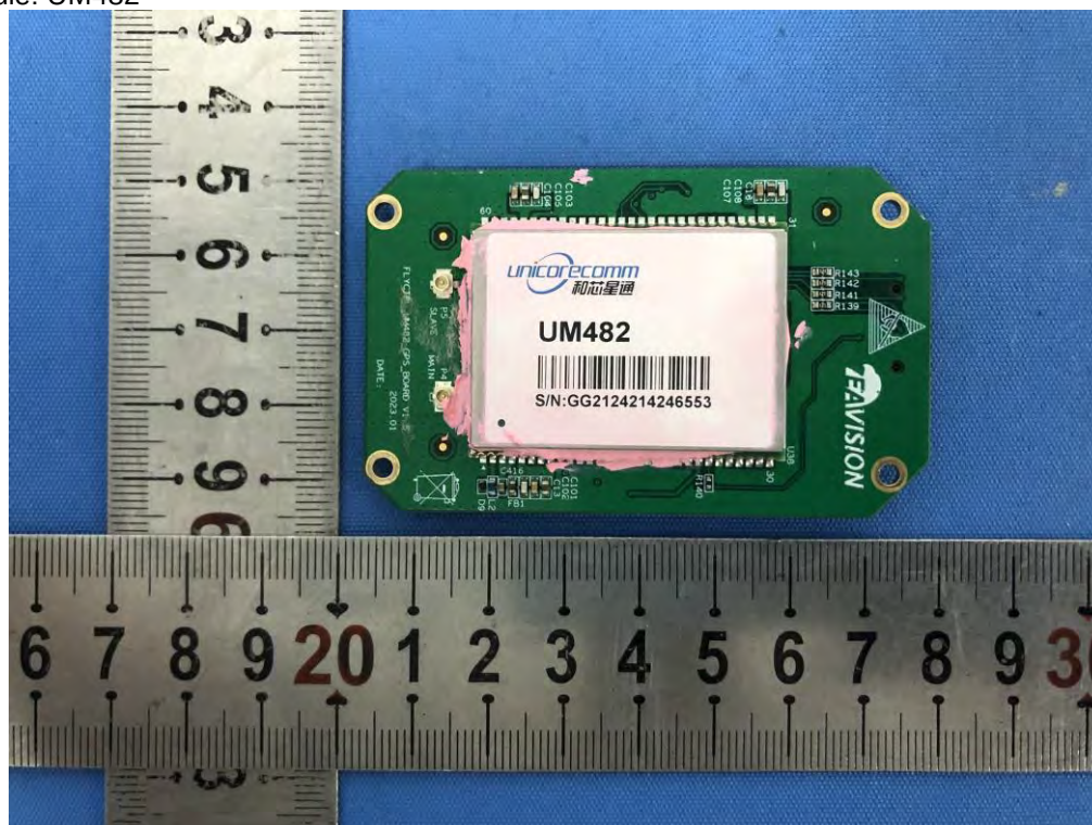
GPS Module: UM482
