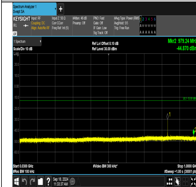
GSM850-190-5-30~1000MHz-PASS
