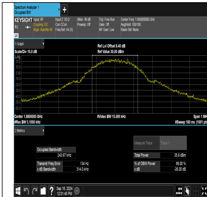
GSM1900-661-0-PASS
