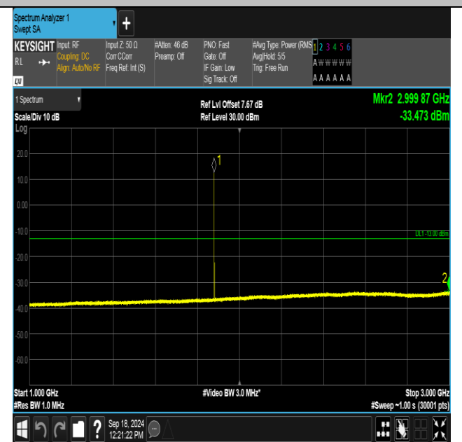
GPRS1900-661-0-1000~3000MHz-PASS
