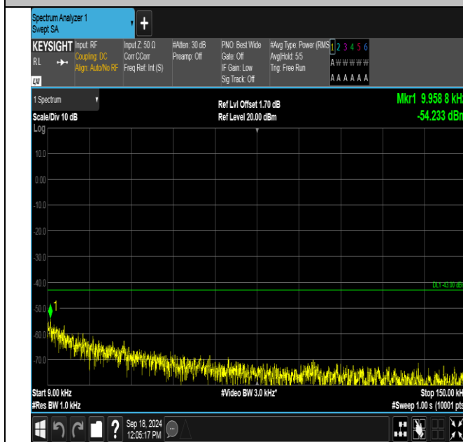
GSM1900-810-0-0.009~0.15MHz-PASS
