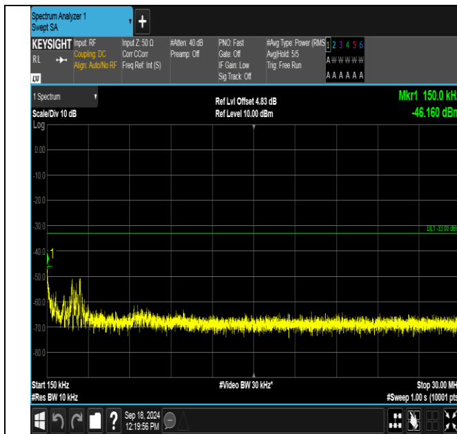
GPRS1900-512-0-0.15~30MHz-PASS
