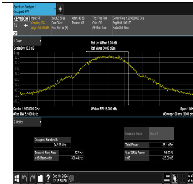
GPRS1900-810-0-PASS
