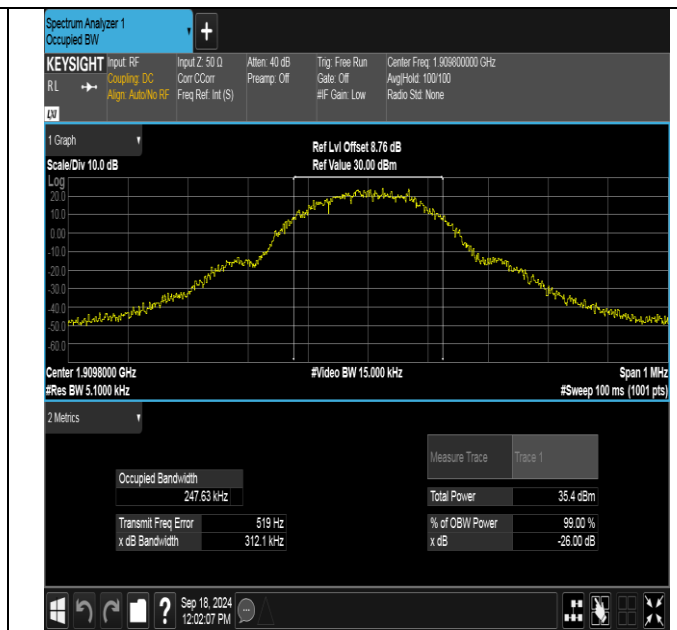
GSM1900-810-0-PASS
