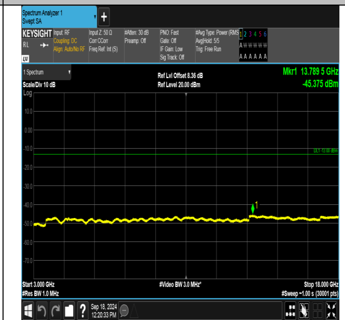
GPRS1900-512-0-3000~18000MHz-PASS
