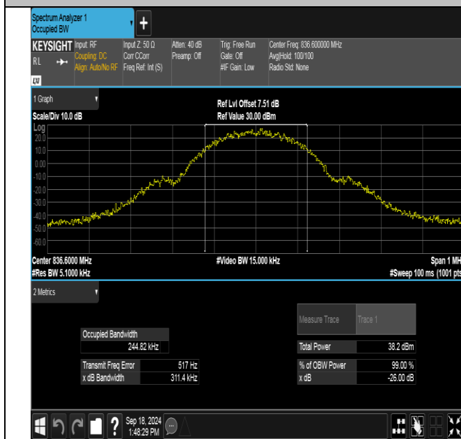
GPRS850-190-5-PASS
