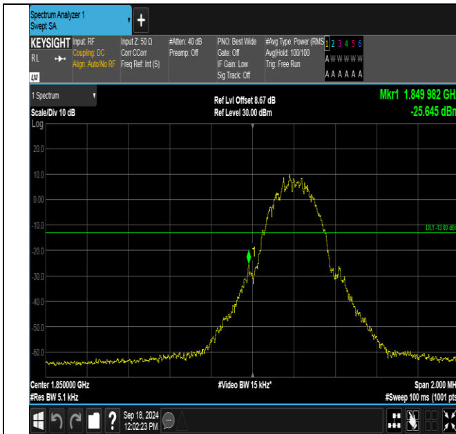
GSM1900-512-0-PASS
