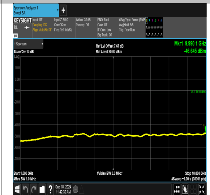
GPRS850-190-5-1000~10000MHz-PASS
