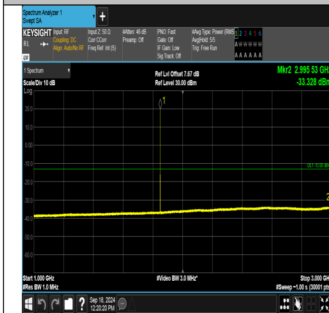
GPRS1900-512-0-1000~3000MHz-PASS
