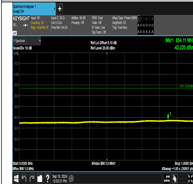
GSM1900-512-0-30~1000MHz-PASS
