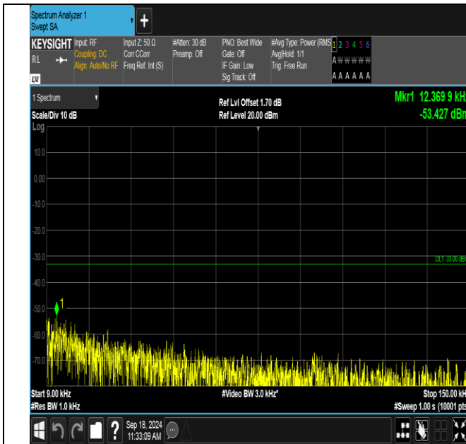
GSM850-190-5-0.009~0.15MHz-PASS
