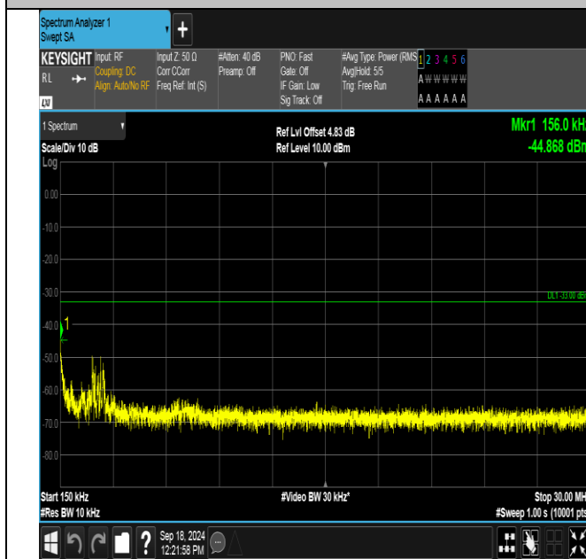
GPRS1900-810-0-0.15~30MHz-PASS
