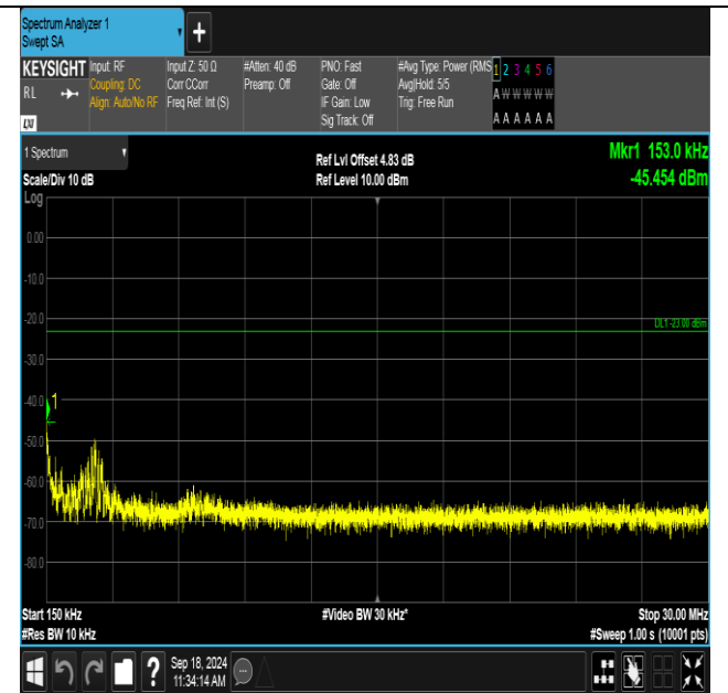
GSM850-251-5-0.15~30MHz-PASS
