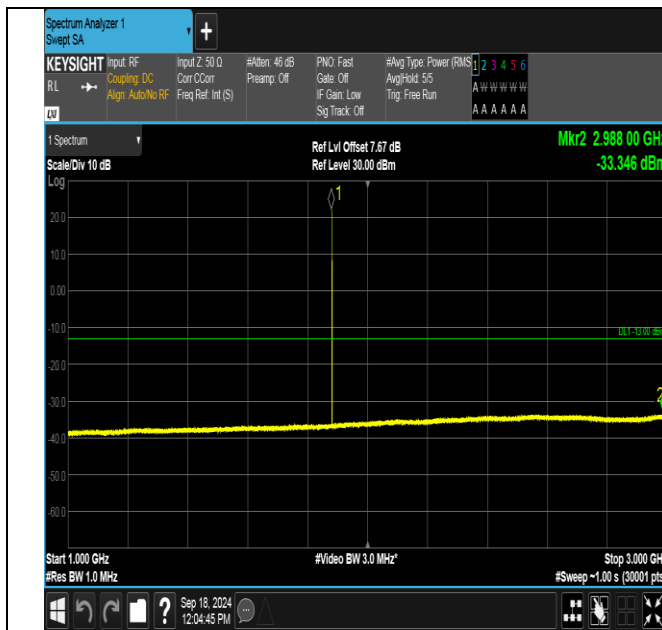
GSM1900-661-0-1000~3000MHz-PASS
