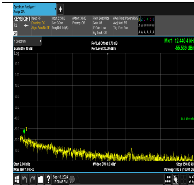
GPRS1900-661-0-0.009~0.15MHz-PASS
