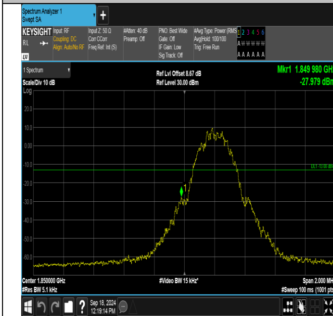
GPRS1900-512-0-PASS
