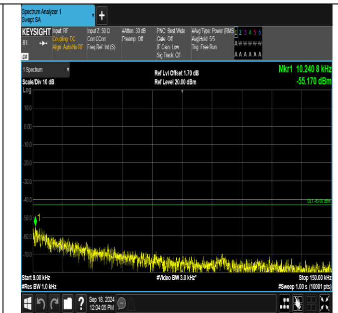
GSM1900-661-0-0.009~0.15MHz-PASS
