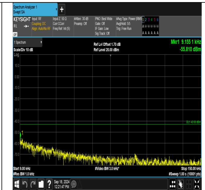
GPRS1900-810-0-0.009~0.15MHz-PASS
