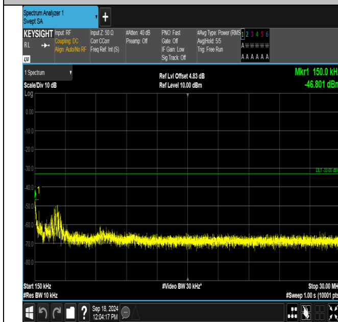
GSM1900-661-0-0.15~30MHz-PASS
