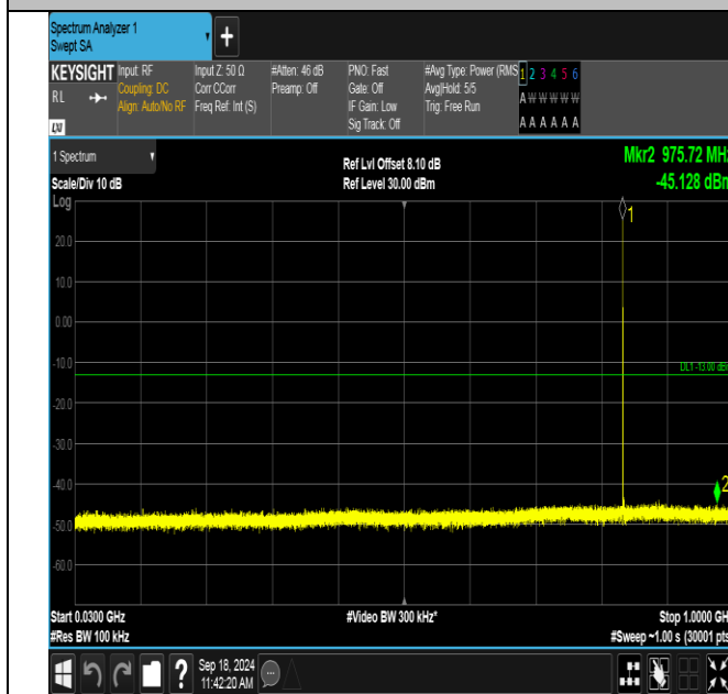
GPRS850-190-5-30~1000MHz-PASS
