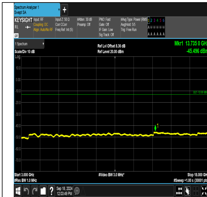
GSM1900-512-0-3000~18000MHz-PASS
