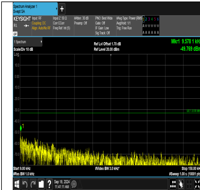
GPRS850-128-5-0.009~0.15MHz-PASS
