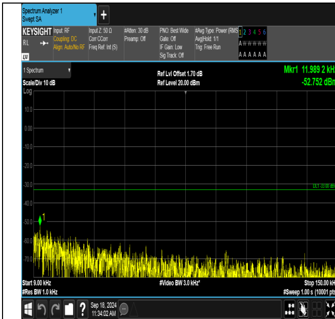
GSM850-251-5-0.009~0.15MHz-PASS
