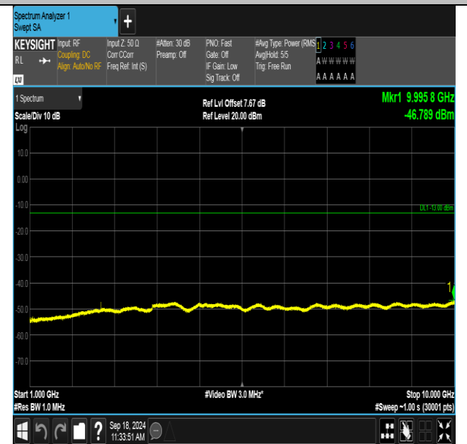
GSM850-190-5-1000~10000MHz-PASS
