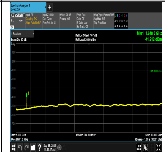
GPRS850-128-5-1000~10000MHz-PASS
