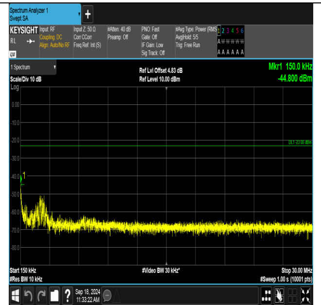
GSM850-190-5-0.15~30MHz-PASS
