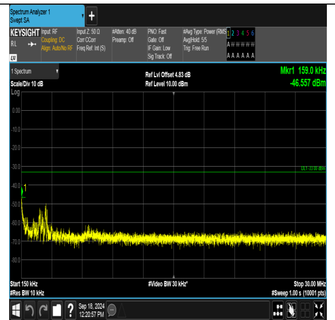
GPRS1900-661-0-0.15~30MHz-PASS
