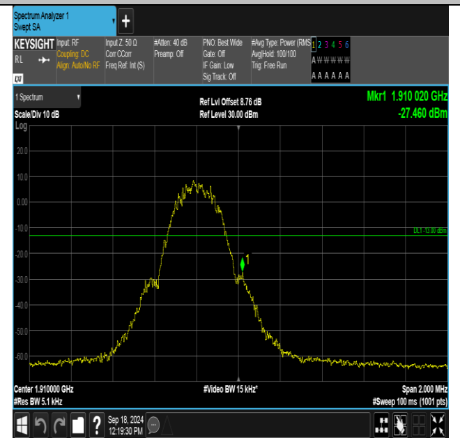
GPRS1900-810-0-PASS
