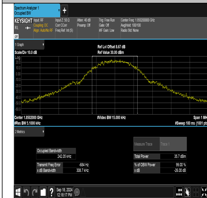
GPRS1900-512-0-PASS
