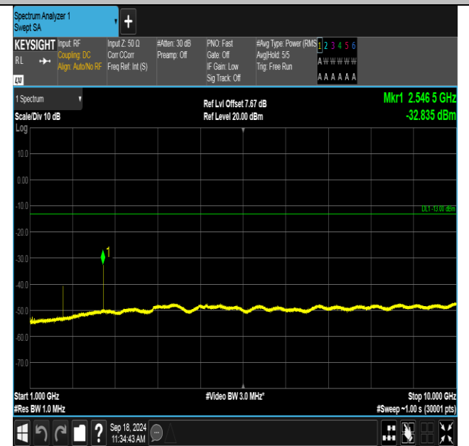
GSM850-251-5-1000~10000MHz-PASS
