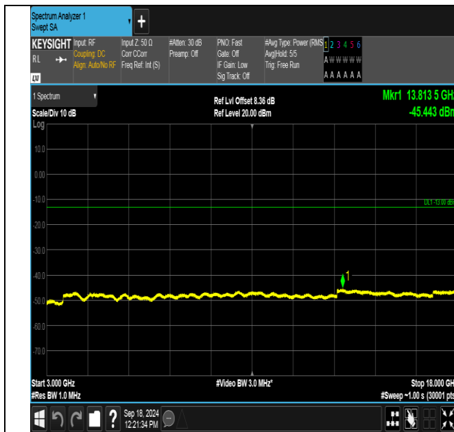
GPRS1900-661-0-3000~18000MHz-PASS
