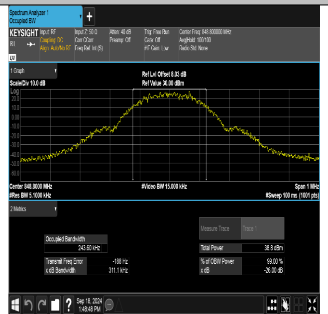
GPRS850-251-5-PASS
