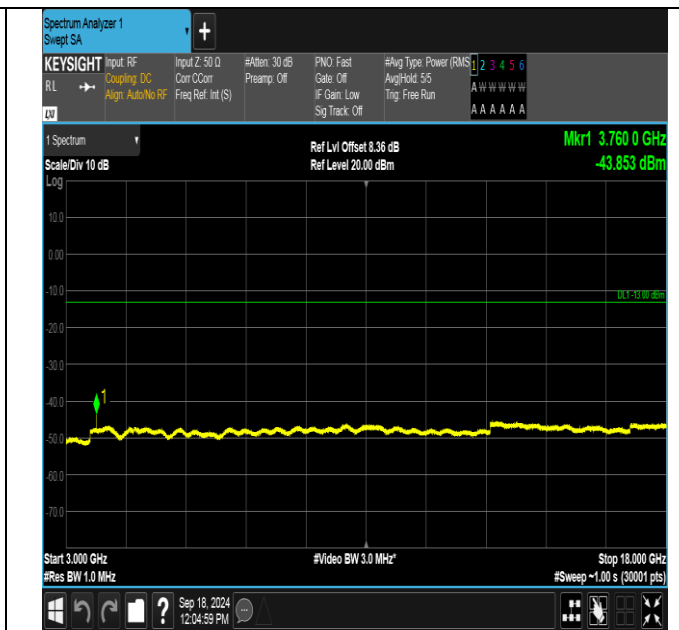
GSM1900-661-0-3000~18000MHz-PASS
