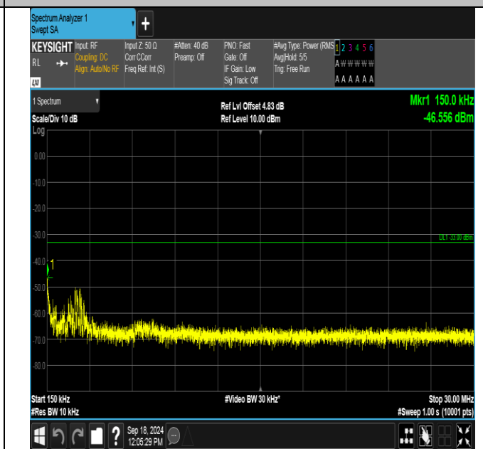
GSM1900-810-0-0.15~30MHz-PASS
