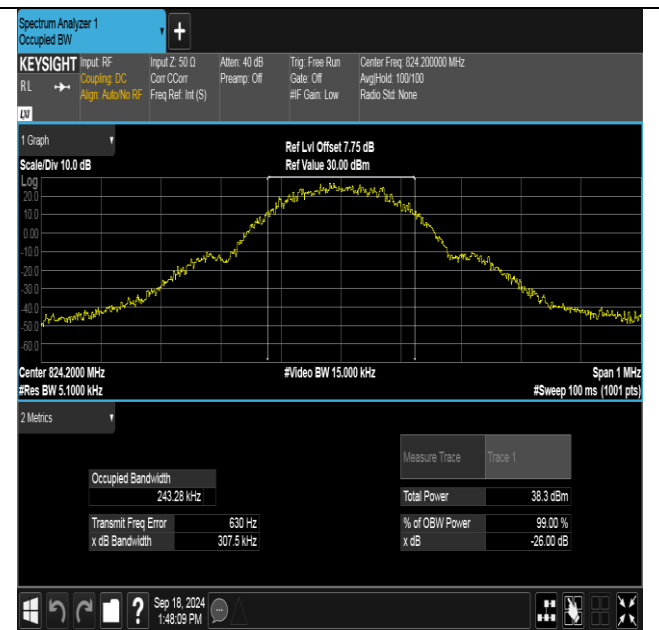
GPRS850-128-5-PASS
