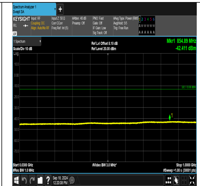
GPRS1900-512-0-30~1000MHz-PASS
