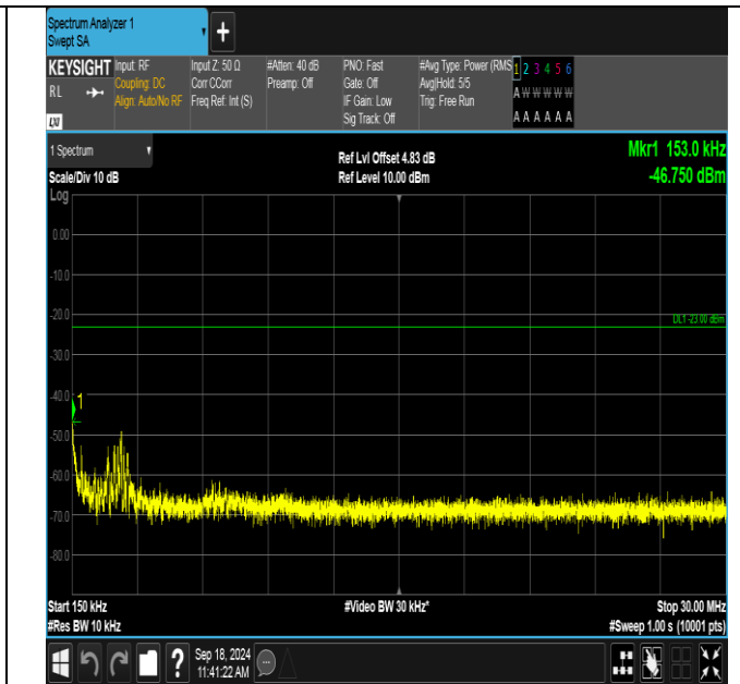
GPRS850-128-5-0.15~30MHz-PASS
