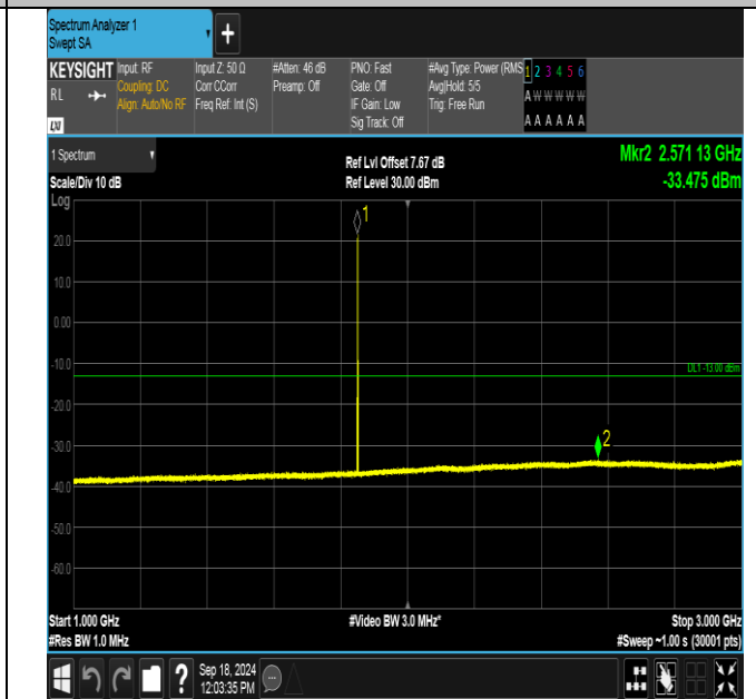
GSM1900-512-0-1000~3000MHz-PASS
