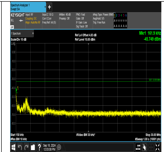
GSM1900-512-0-0.15~30MHz-PASS
