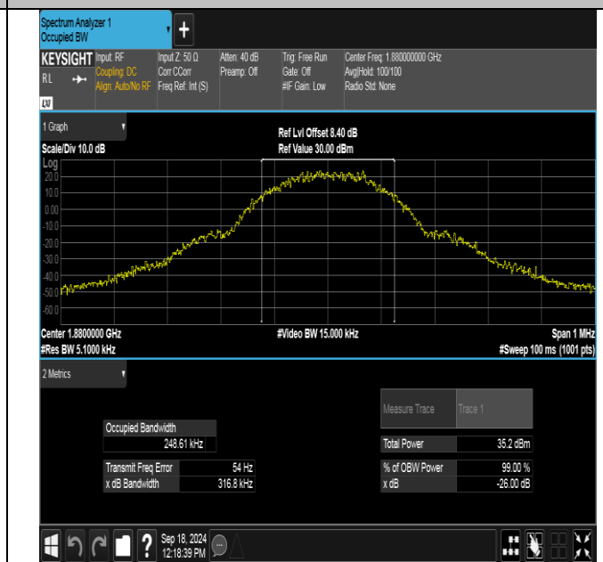
GPRS1900-661-0-PASS
