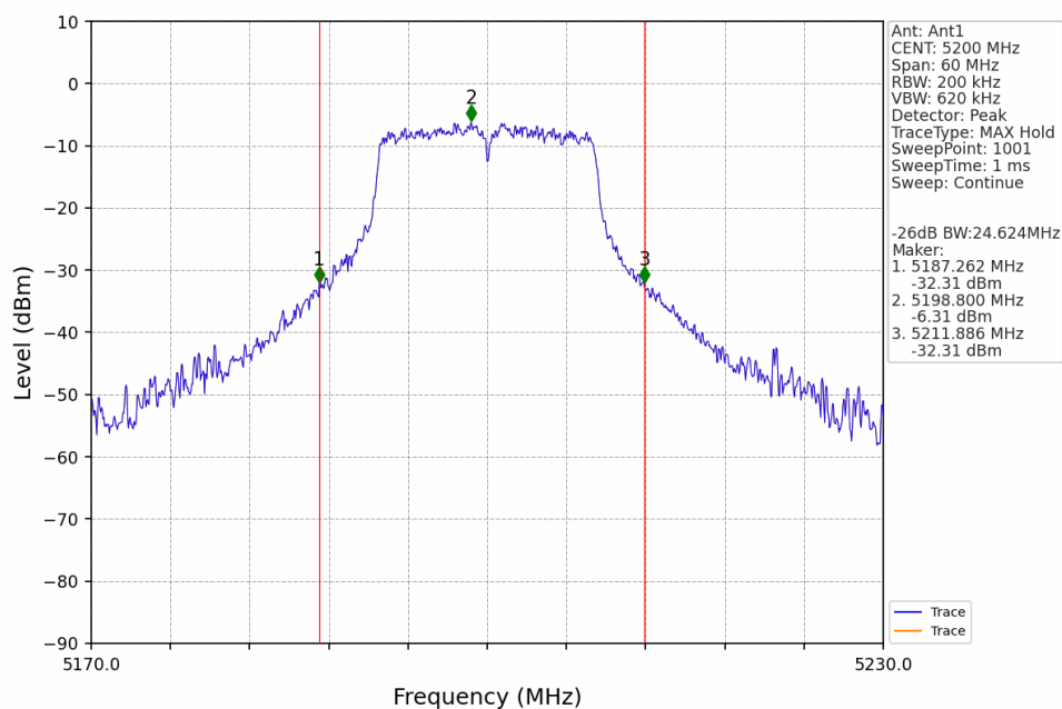
802.11a_MCH_5200MHz_Ant1_NTNV
