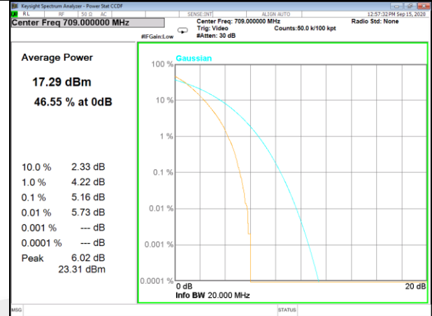
Band17_50_Q16_Low
