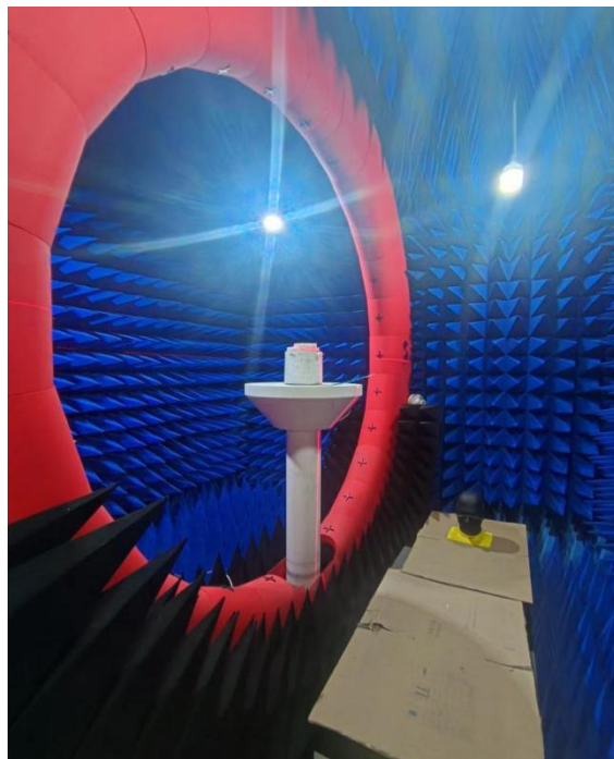
暗室内部 Inside the ETS anechoic chamber
