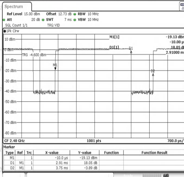
NTNV-2DH5-Ant1-2480
