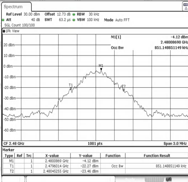
DH5-Ant1-2480
