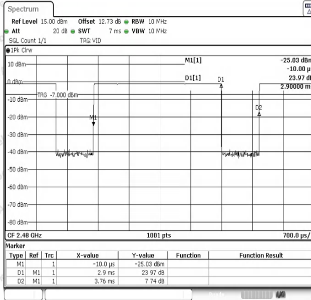
NTNV-DH5-Ant1-2480
