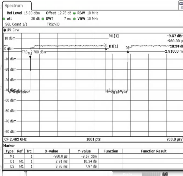
NTNV-2DH5-Ant1-2402
