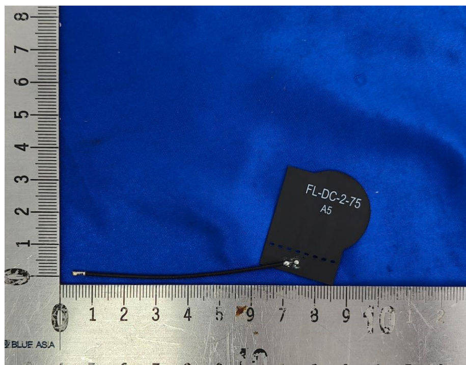
Ant5: FL-DC-2-75
