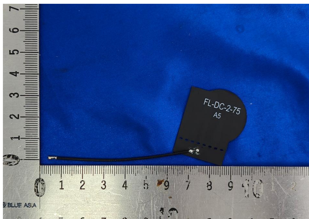
Ant5: FL-DC-2-75
