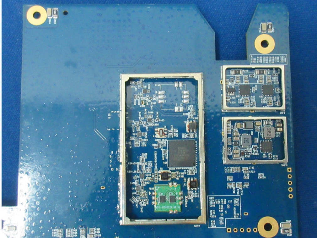
(62) EUT Photo
