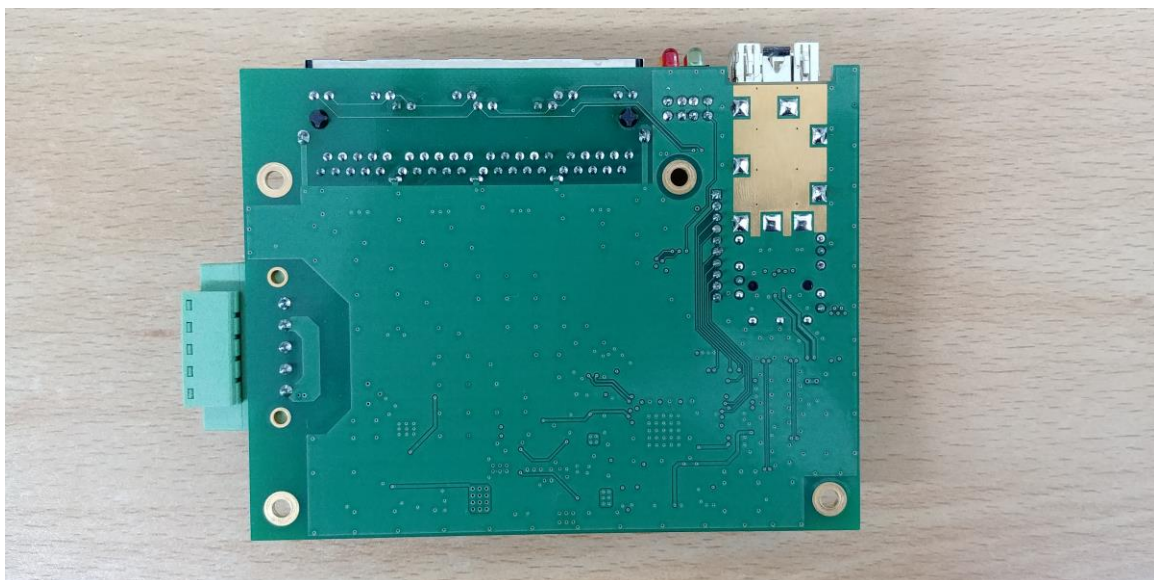
MDC_bottom
