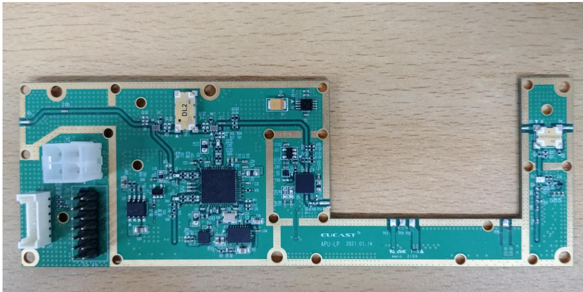
APU_LP_top
