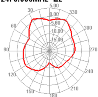
2475.000MHz E2
