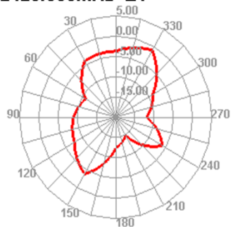
2425.000MHz E1
