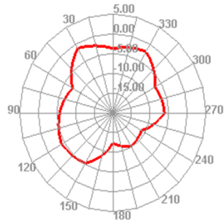
2425.000MHz E2
