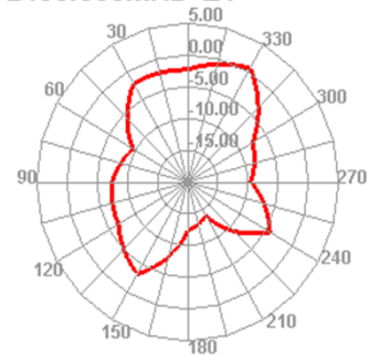
2450.000MHz E1
