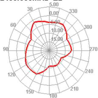
2400.000MHz E2
