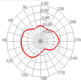
2425.000MHz H
