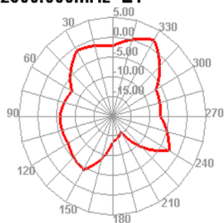
2500.000MHz E1
