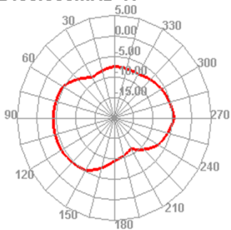
2450.000MHz E2
