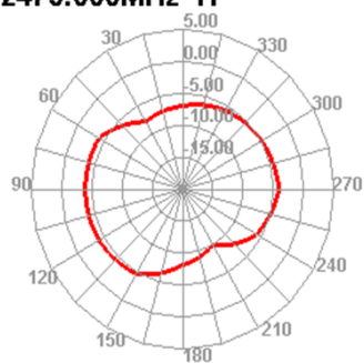
2475.000MHz H
