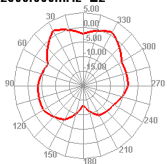
2500.000MHz E2
