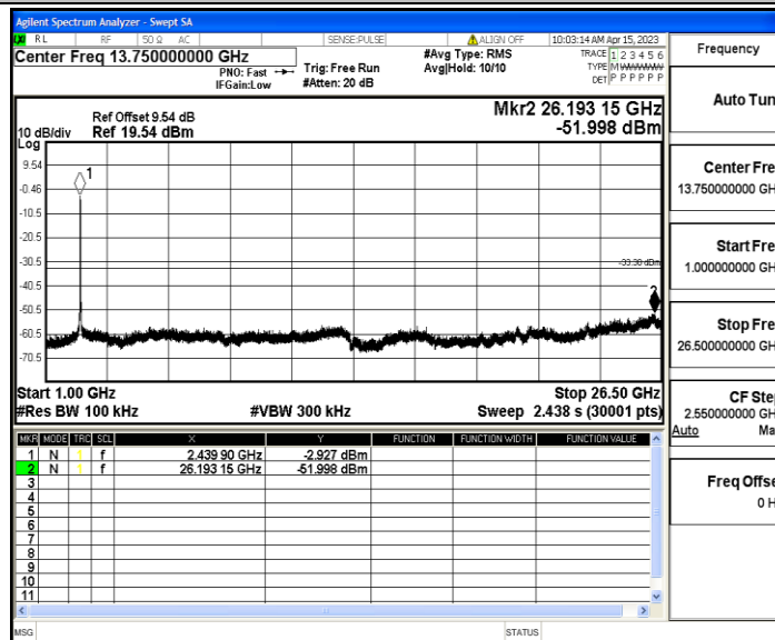
11N40MIMO_Ant2_2452_1000~26500
