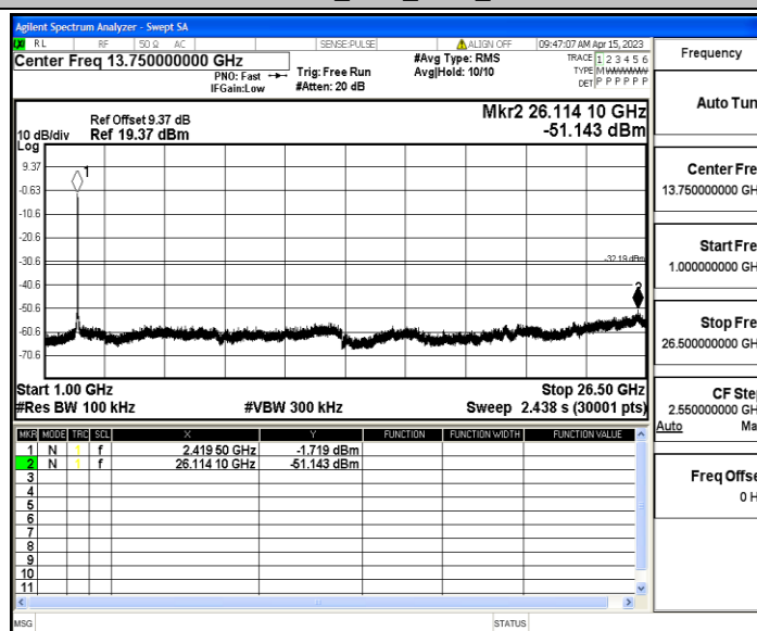
11N40MIMO_Ant2_2422_1000~26500
