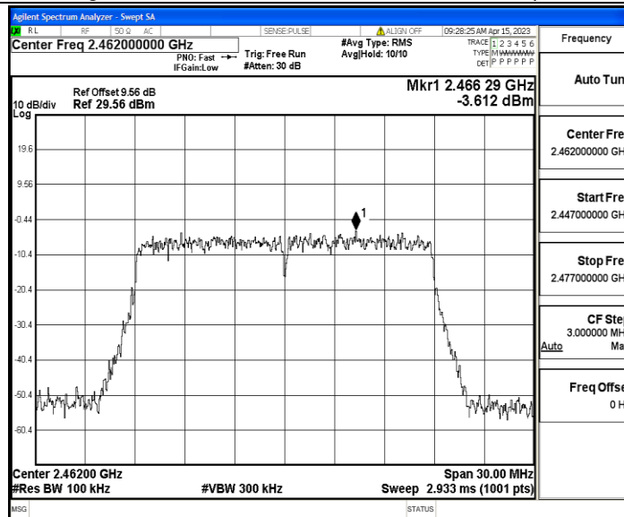
11N20MIMO_Ant1_2462_0~Reference
