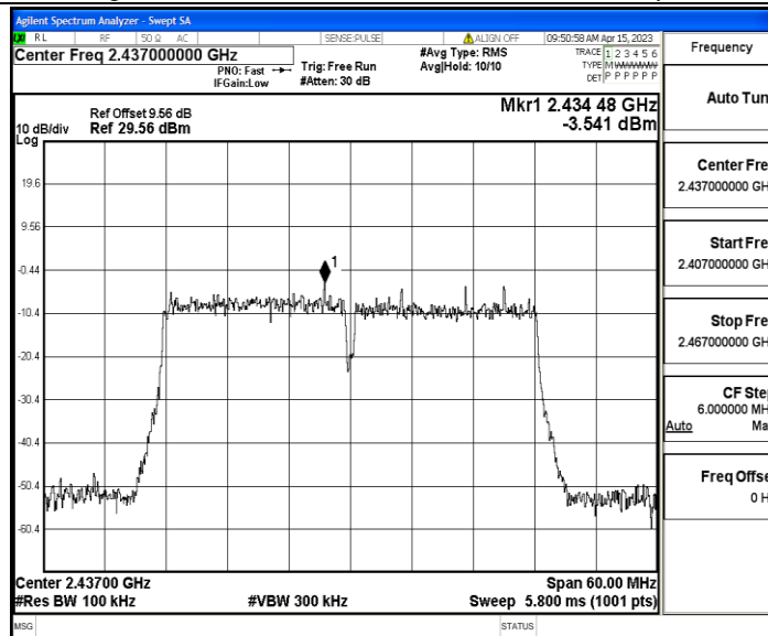
11N40MIMO_Ant1_2437_0~Reference
