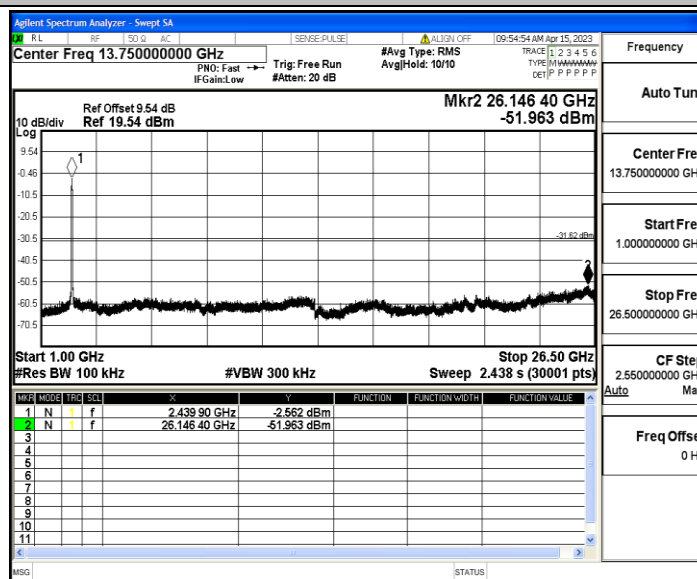
11N40MIMO_Ant2_2437_1000~26500
