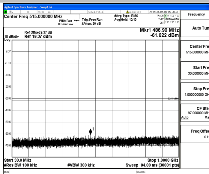
11N40MIMO_Ant2_2422_30~1000
