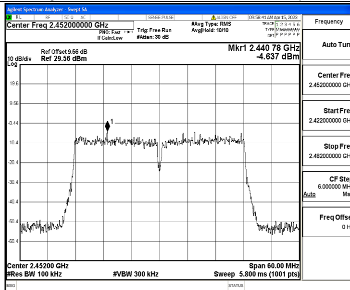
11N40MIMO_Ant1_2452_0~Reference
