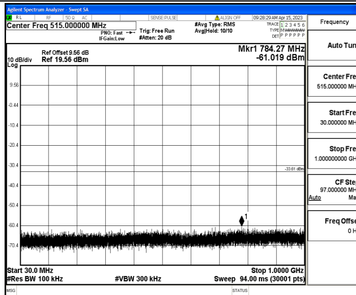
11N20MIMO_Ant1_2462_30~1000
