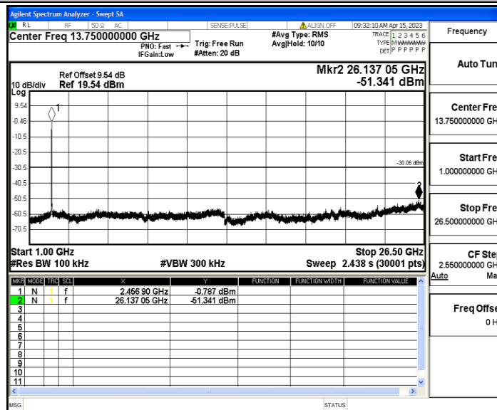
11N20MIMO_Ant2_2462_1000~26500
