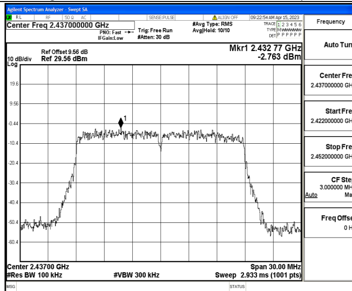
11N20MIMO_Ant1_2437_0~Reference
