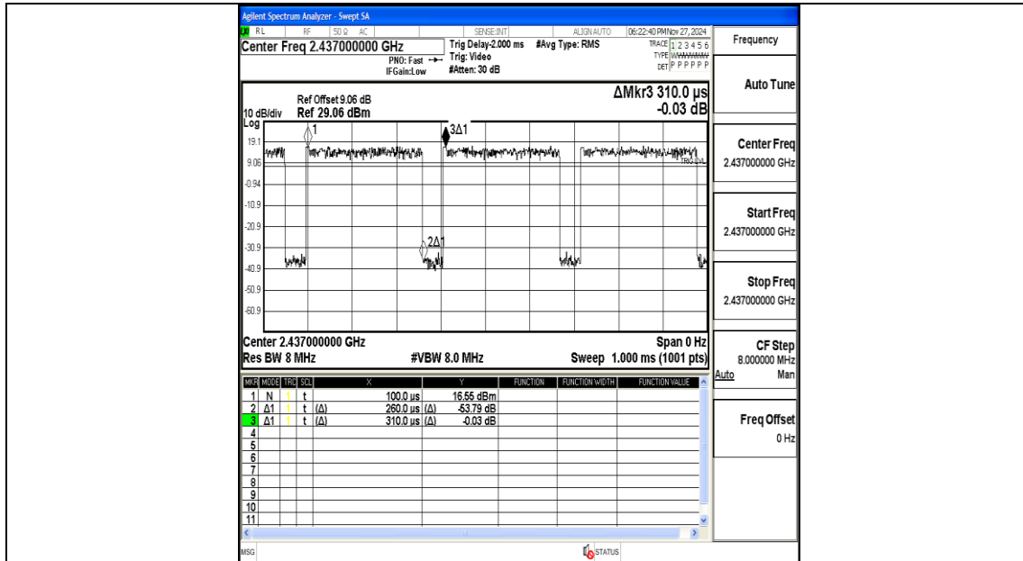
NTNV-11AX20MIMO-Ant1-2437
