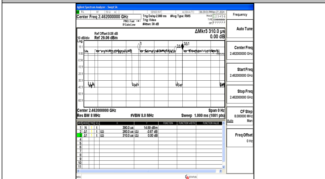
NTNV-11AX20MIMO-Ant1-2462
