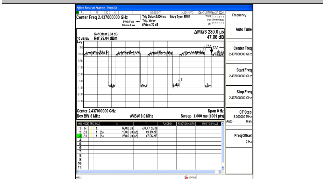
NTNV-11AX40MIMO-Ant2-2437
