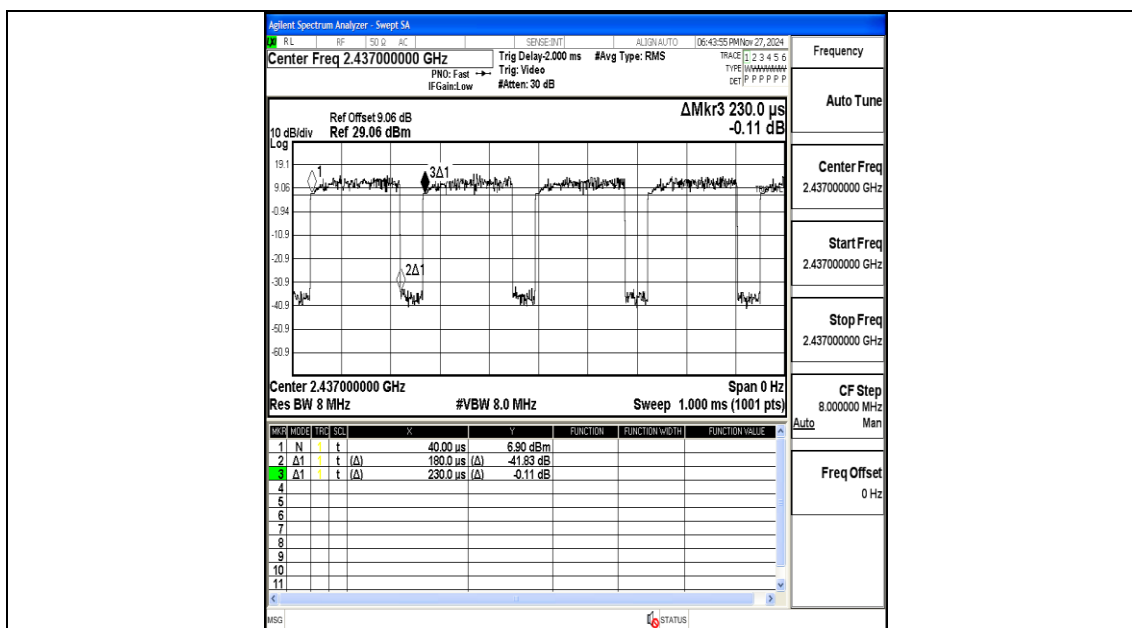
NTNV-11AX40MIMO-Ant1-2437
