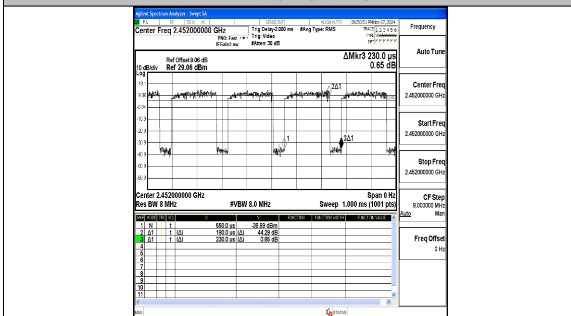
NTNV-11AX40MIMO-Ant1-2452
