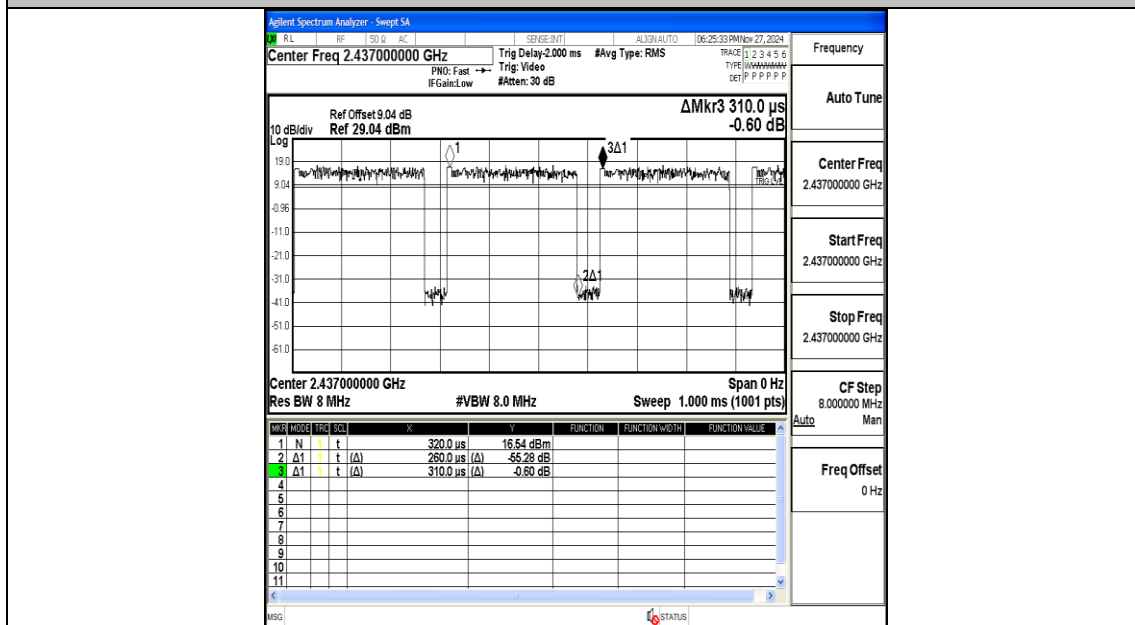
NTNV-11AX20MIMO-Ant2-2437
