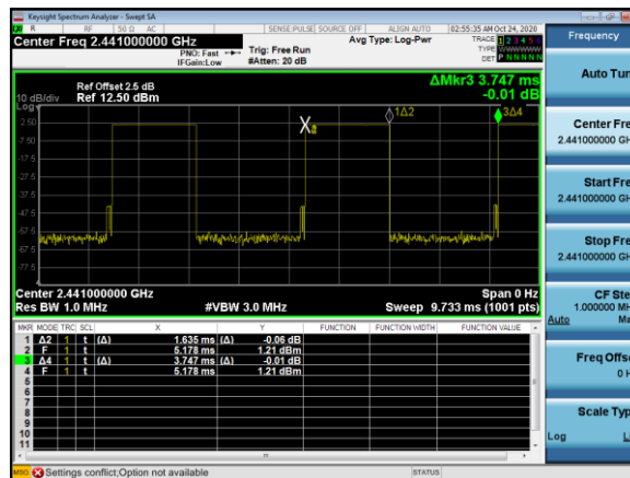
DH3
