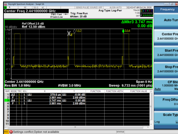
DH1
