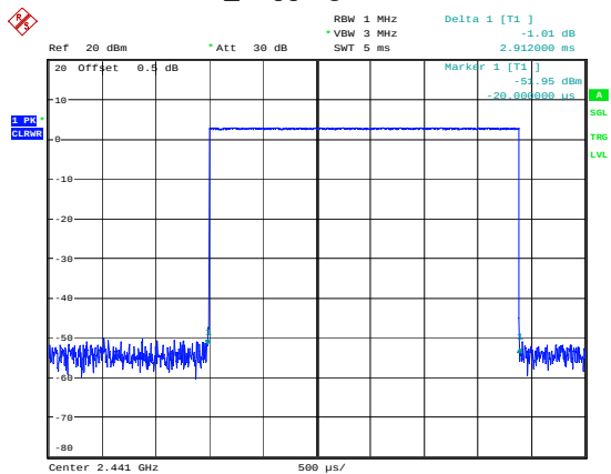
DH5_Hopping 2.912ms
