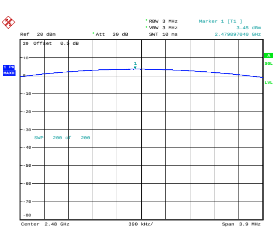
DH1_2480 3.45dBm
