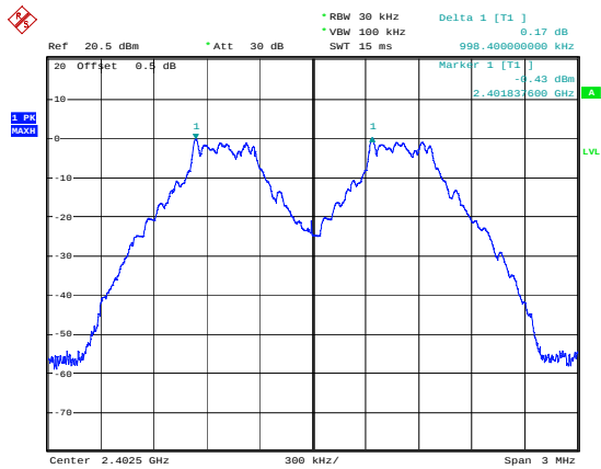
DH1_Low 0.998MHz
