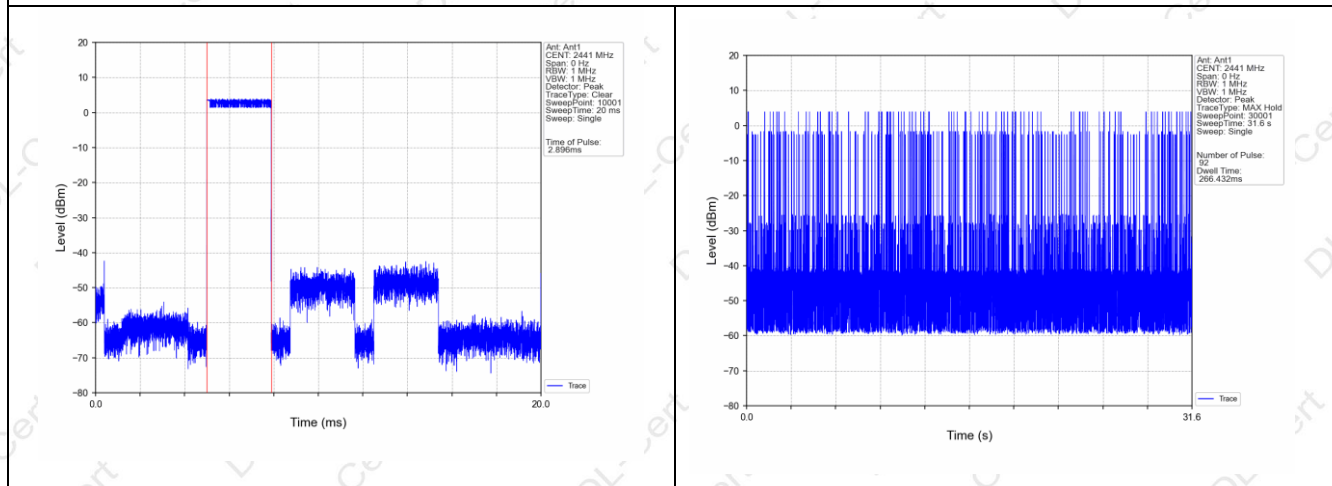
2-DH5
