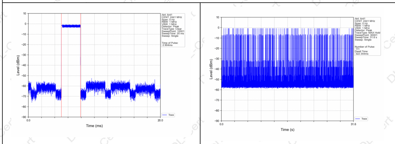
3-DH5
