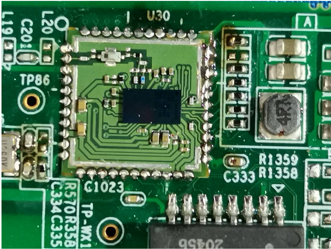
Zigbee Module
