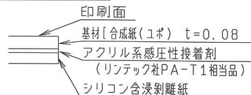
材料構成図
