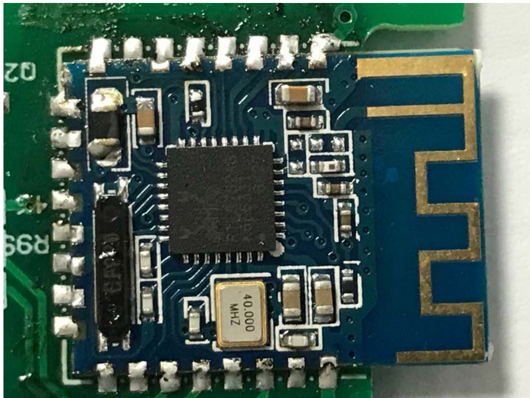
BLE Module
