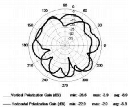
SN01—EUT vertical
