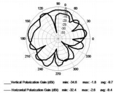
SN02—EUT side
