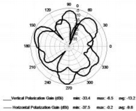
SN01—EUT side
