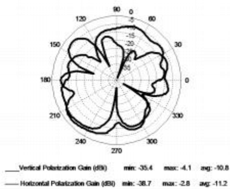
SN01—EUT vertical
