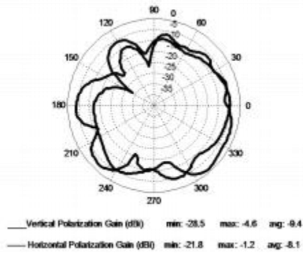
SN01—EUT side
