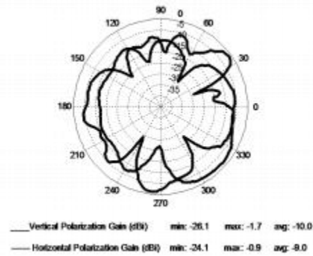
SN02—EUT side
