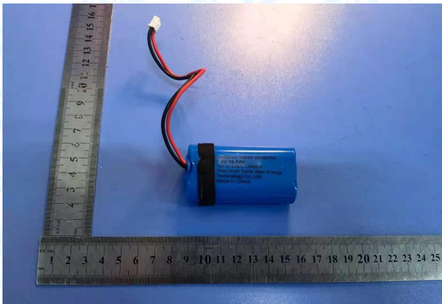
Photo 23 Battery Parameters
