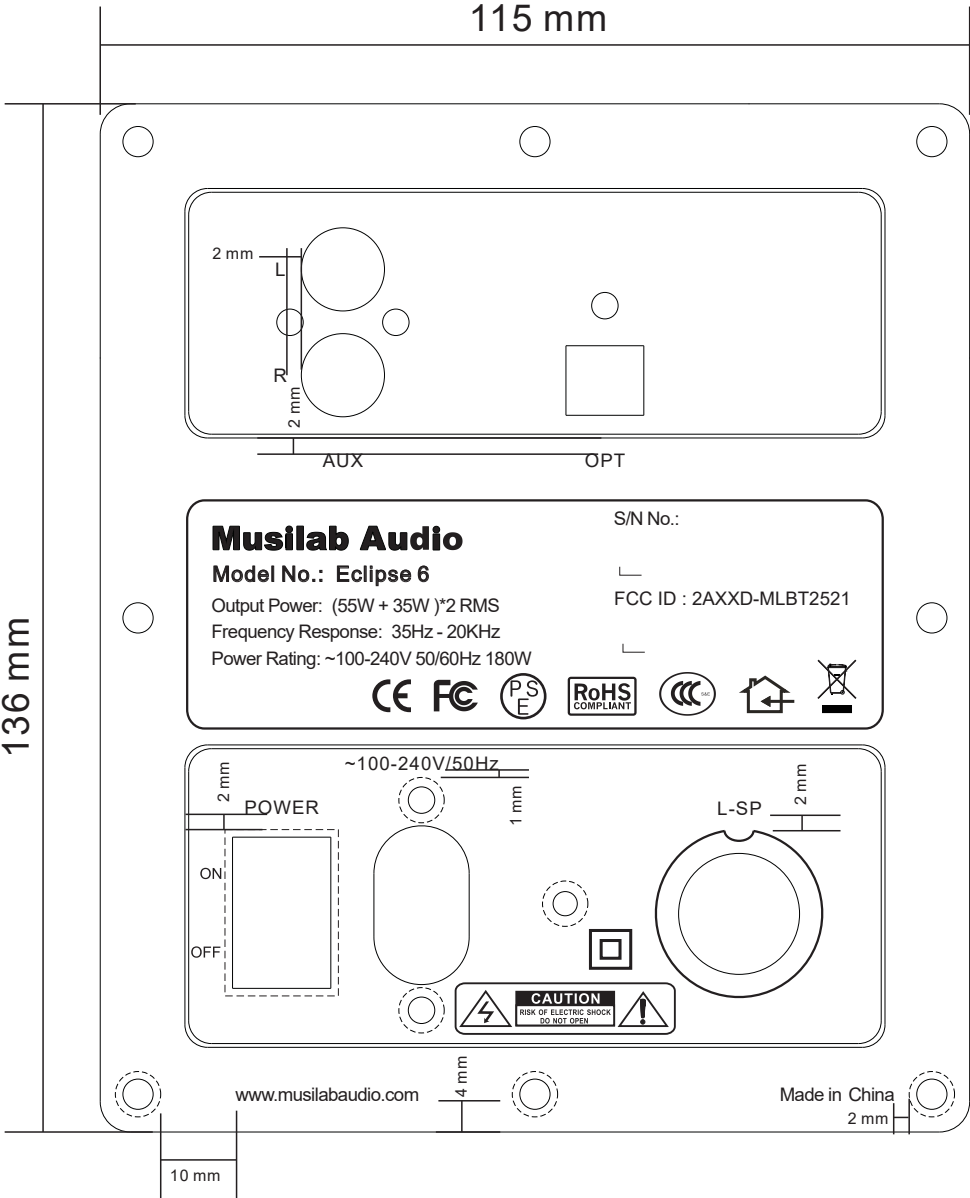
主机后板丝印参照图
