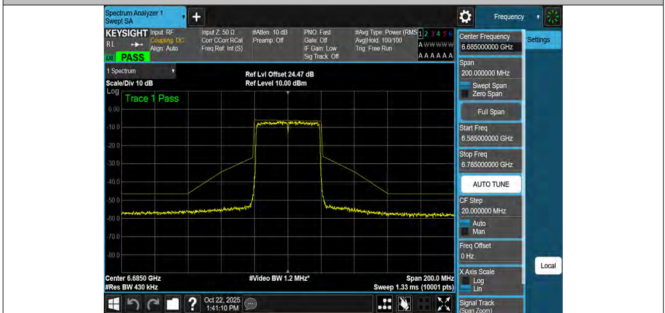
NTNV-11AX40MIMO-Ant4-6685-PASS
