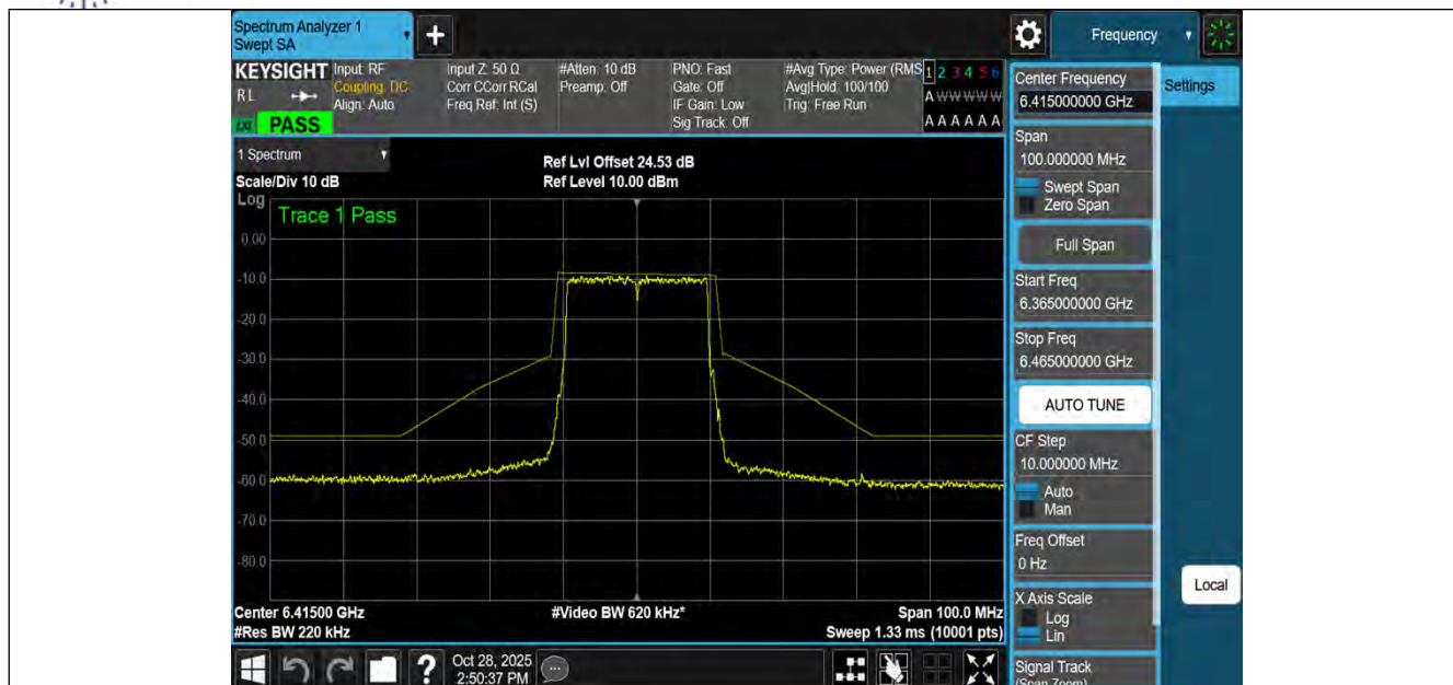
NTNV-11BE20MIMO-Ant1-6415-PASS
