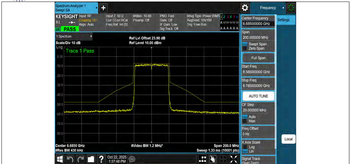
NTNV-11AX40MIMO-Ant1-6685-PASS
