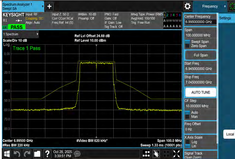
NTNV-11BE20MIMO-Ant1-6995-PASS
