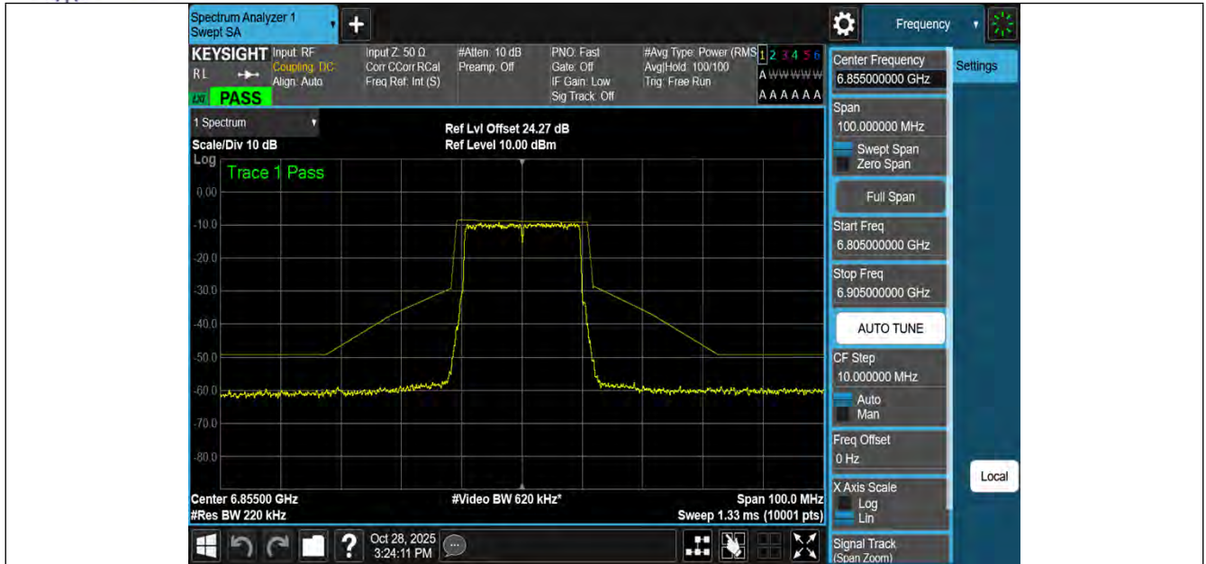
NTNV-11BE20MIMO-Ant1-6855-PASS
