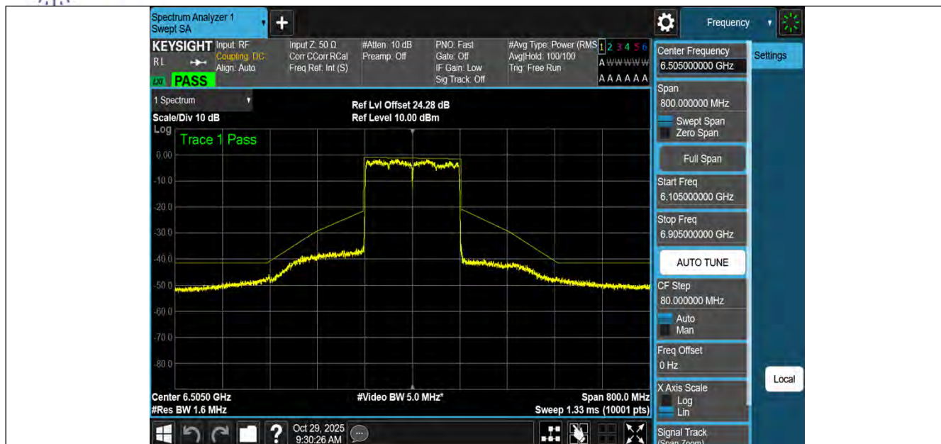
NTVN-11BE160MIMO-Ant1-6505-PASS
