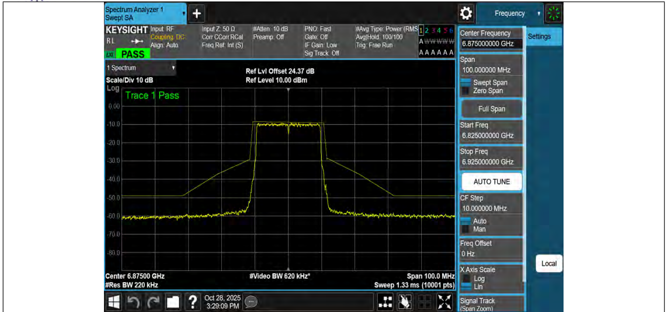
NTNV-11BE20MIMO-Ant1-6875-PASS
