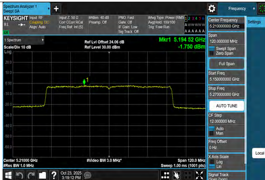
11AX80MIMO-Ant1-5210-PASS
