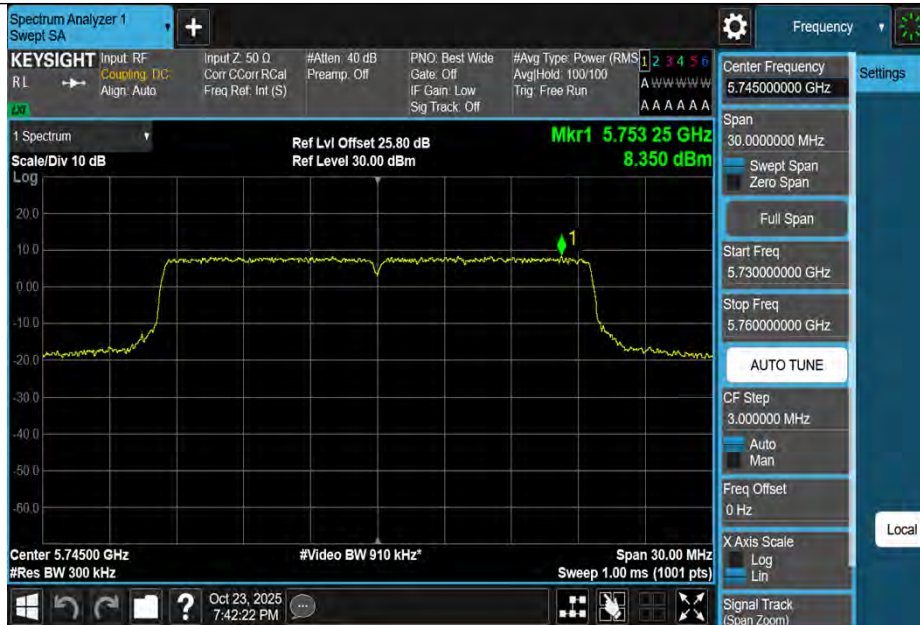
11AX20MIMO-Ant1-5745-PASS
