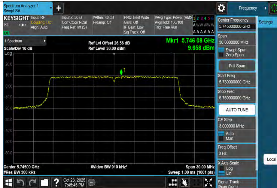
11AX20MIMO-Ant3-5745-PASS
