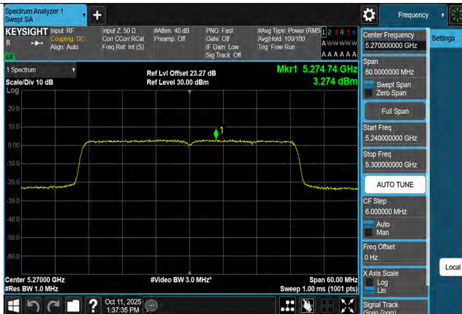
11AX40MIMO-Ant1-5270-PASS
