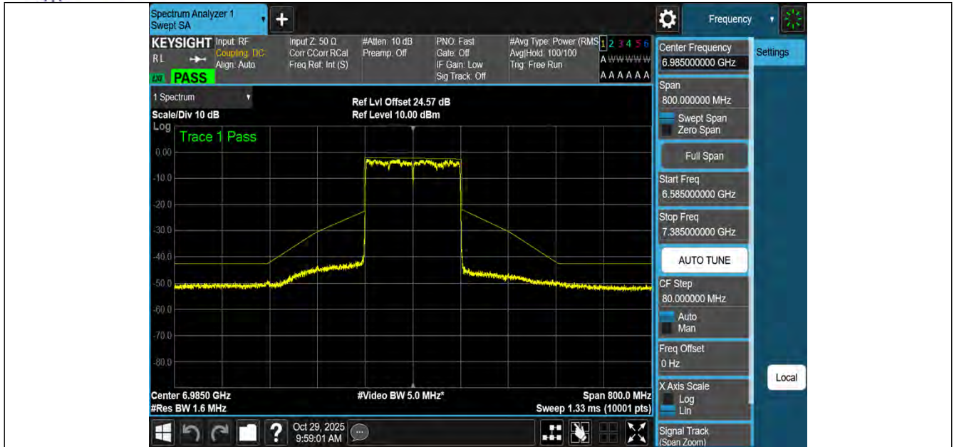
NTVN-11BE160MIMO-Ant1-6985-PASS
