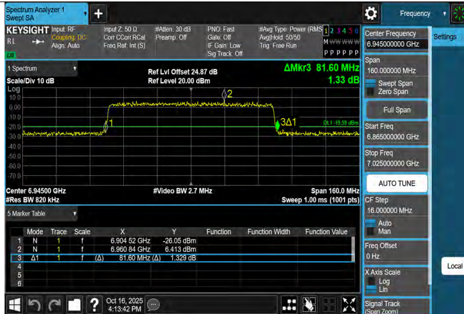
11AX80MIMO-Ant3-6945
