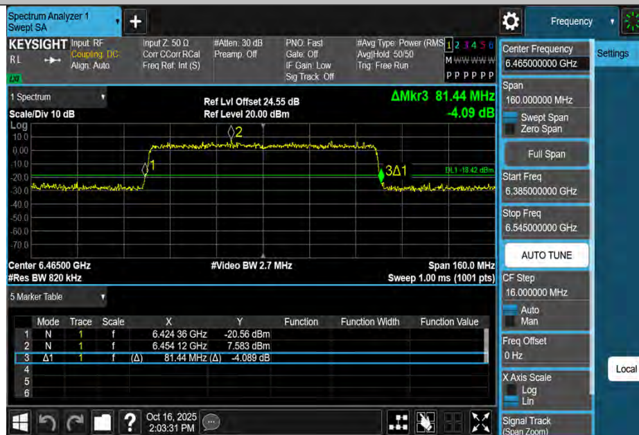
11AX80MIMO-Ant4-6465
