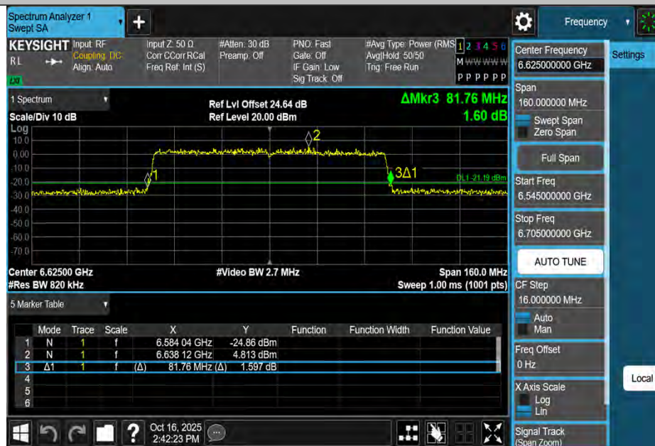
11AX80MIMO-Ant4-6625
