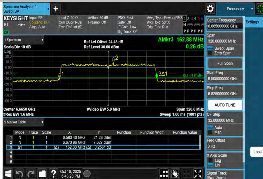
11AX160MIMO-Ant4-6665
