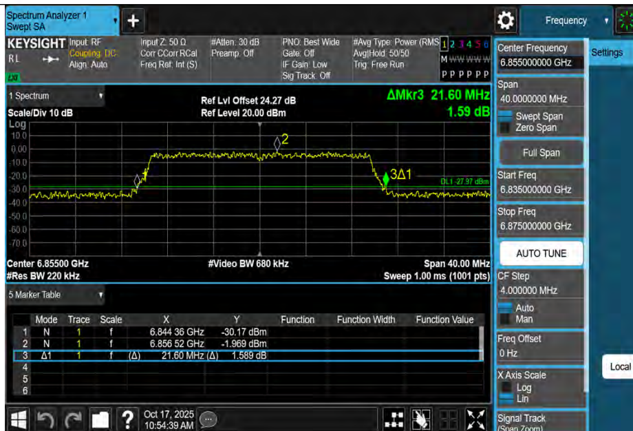
11BE20MIMO-Ant1-6855
