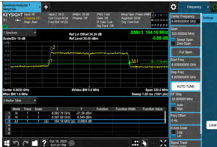
11AX160MIMO-Ant1-6665
