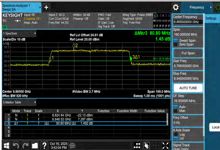
11AX80MIMO-Ant4-6865
