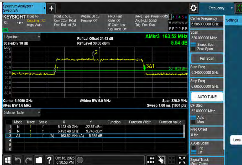
11AX160MIMO-Ant4-6505
