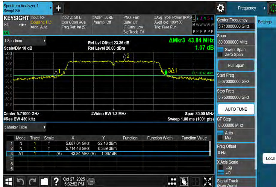
11N40MIMO-Ant1-5710
