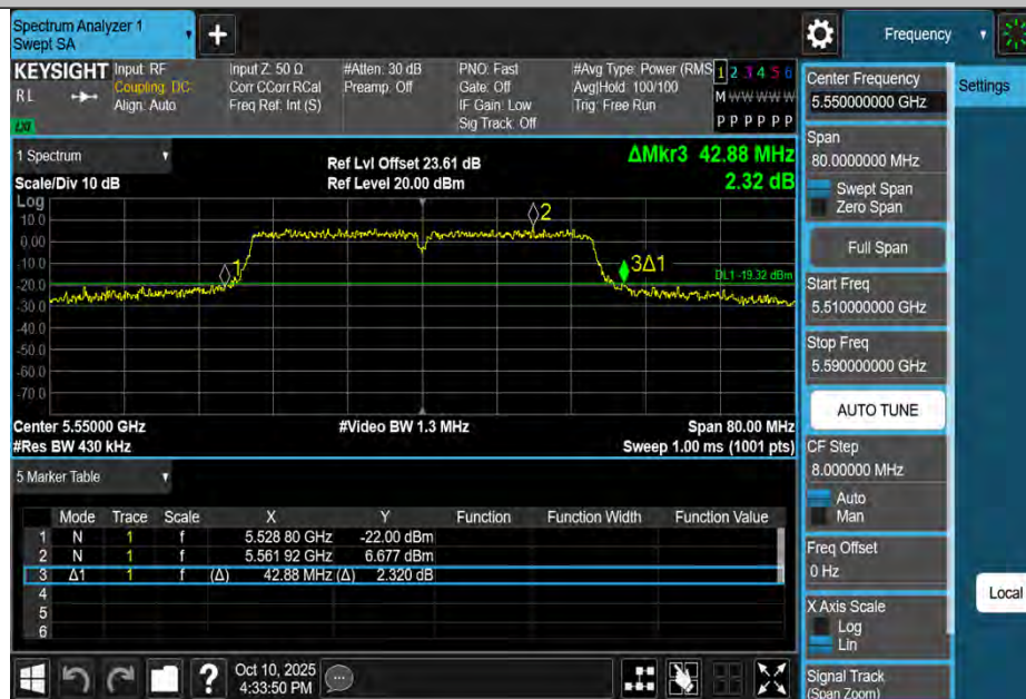
11AC40MIMO-Ant1-5550
