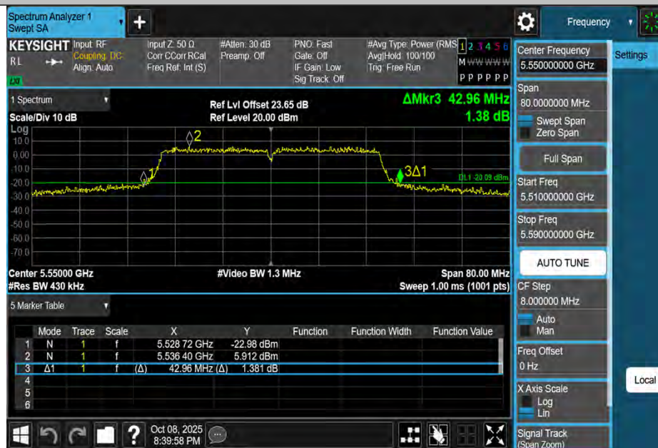
11N40MIMO-Ant3-5550
