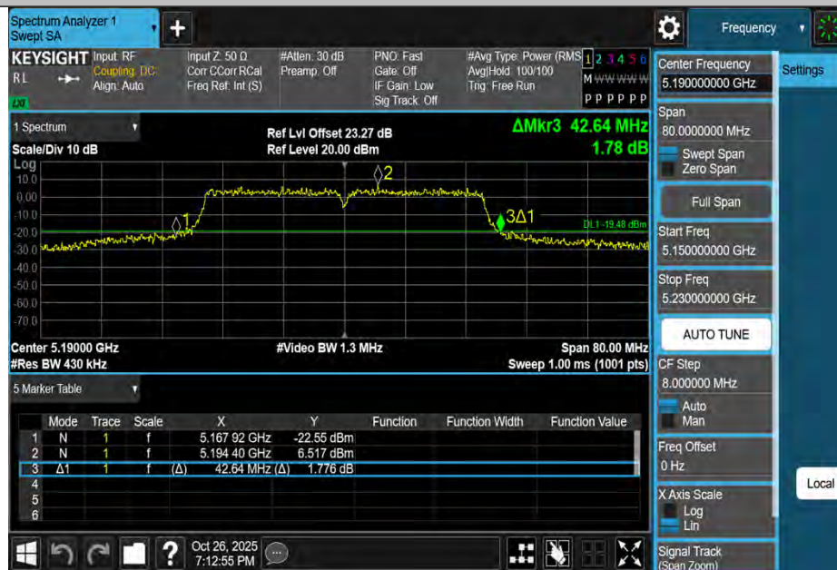
11N40MIMO-Ant1-5190
