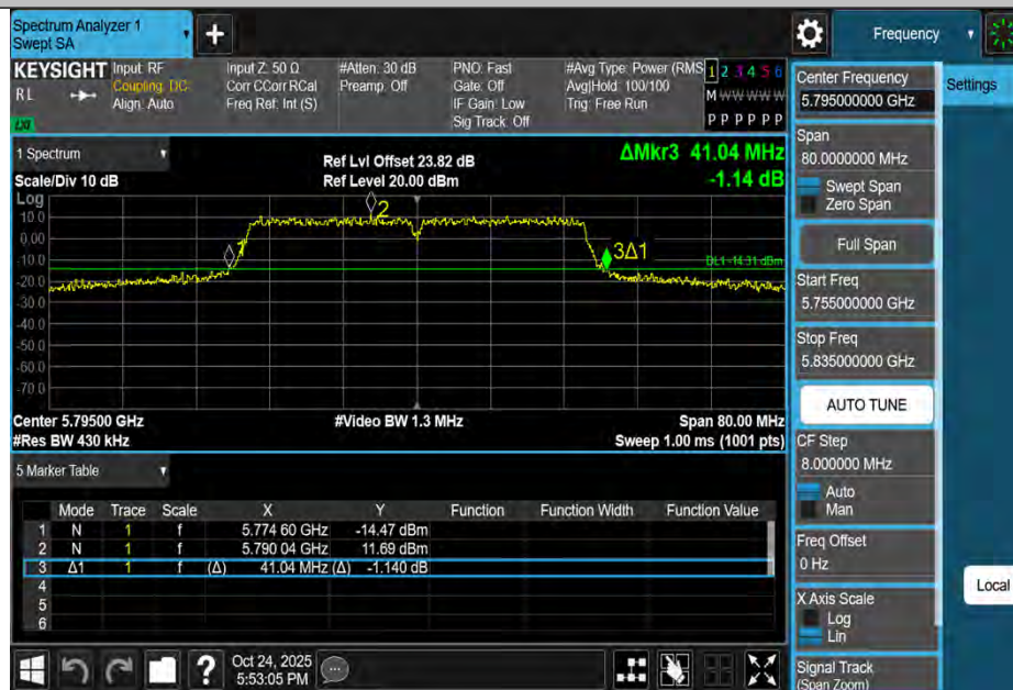
11N40MIMO-Ant2-5795
