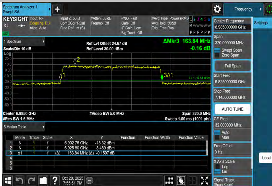
11BE160MIMO-Ant4-6985
