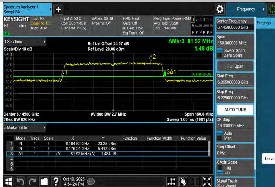
11BE80MIMO-Ant4-6145
