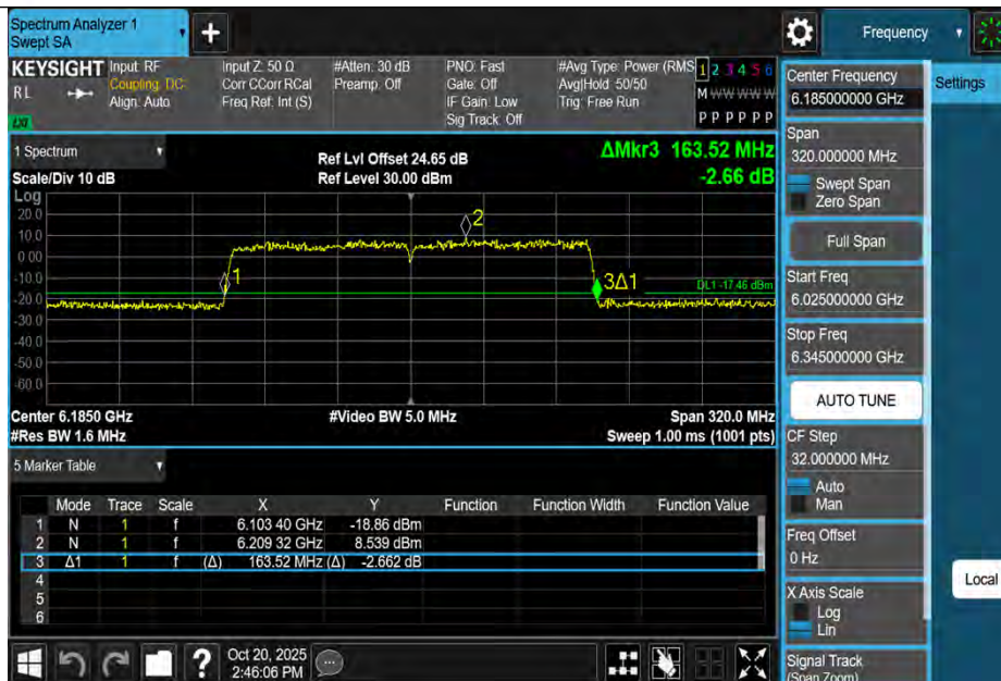
11BE160MIMO-Ant3-6185
