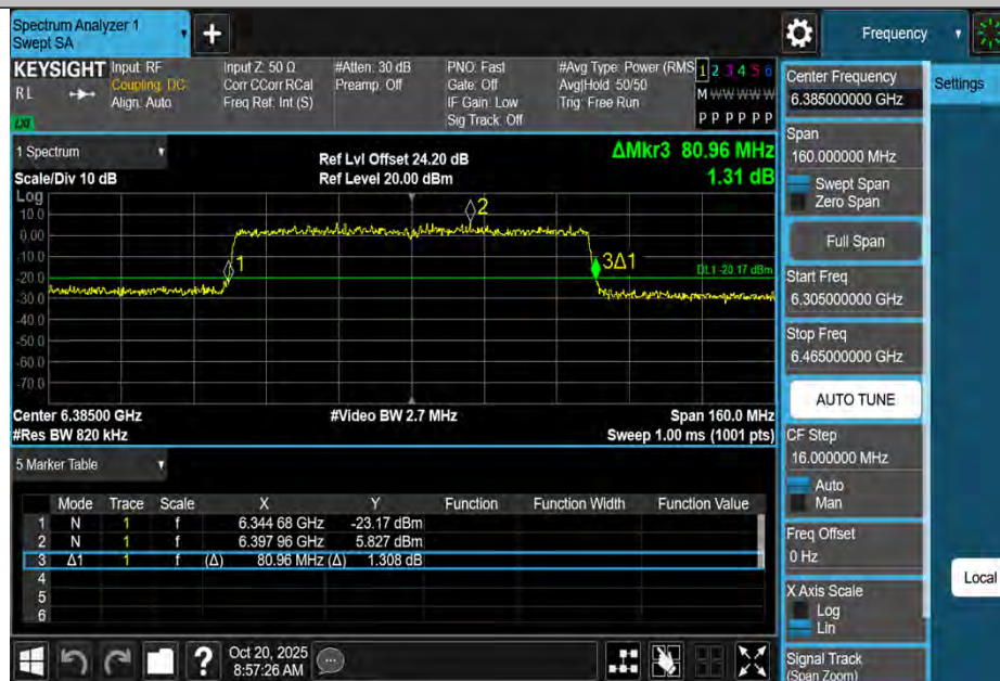
11BE80MIMO-Ant4-6385
