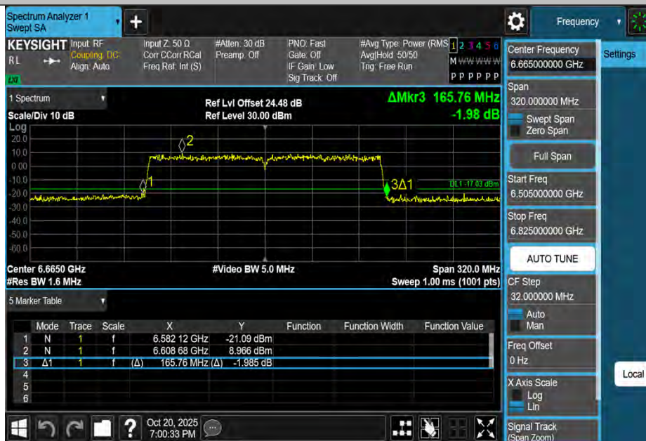
11BE160MIMO-Ant4-6665
