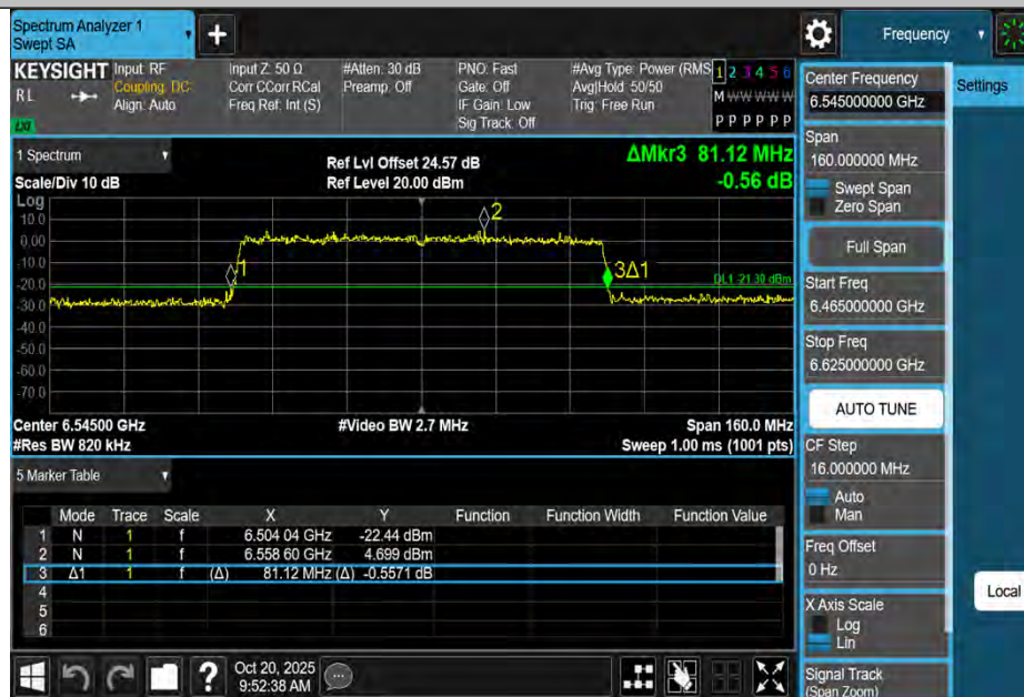
11BE80MIMO-Ant4-6545
