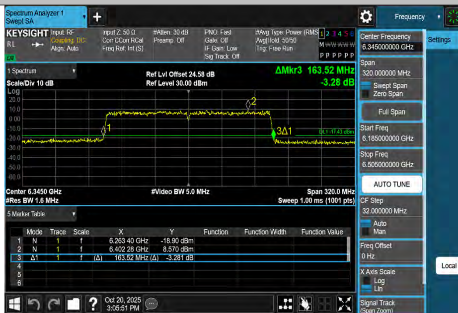
11BE160MIMO-Ant4-6345
