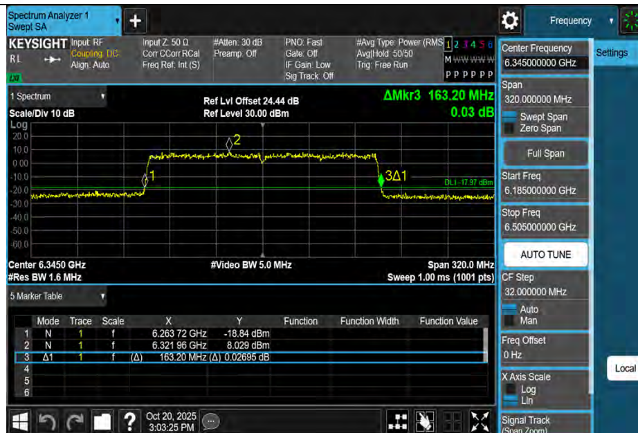
11BE160MIMO-Ant3-6345
