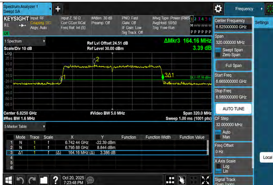
11BE160MIMO-Ant1-6825
