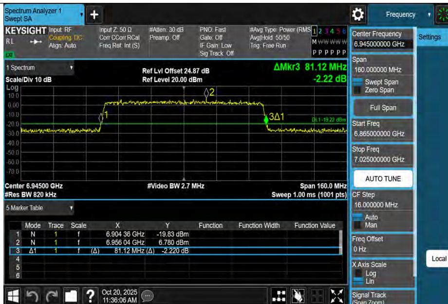
11BE80MIMO-Ant3-6945
