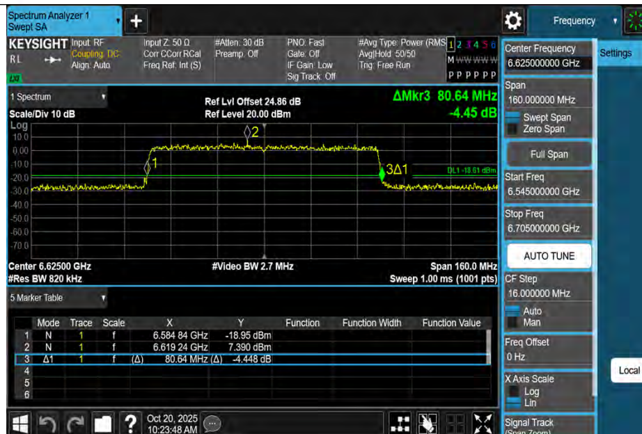
11BE80MIMO-Ant3-6625
