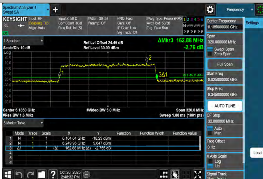
11BE160MIMO-Ant4-6185
